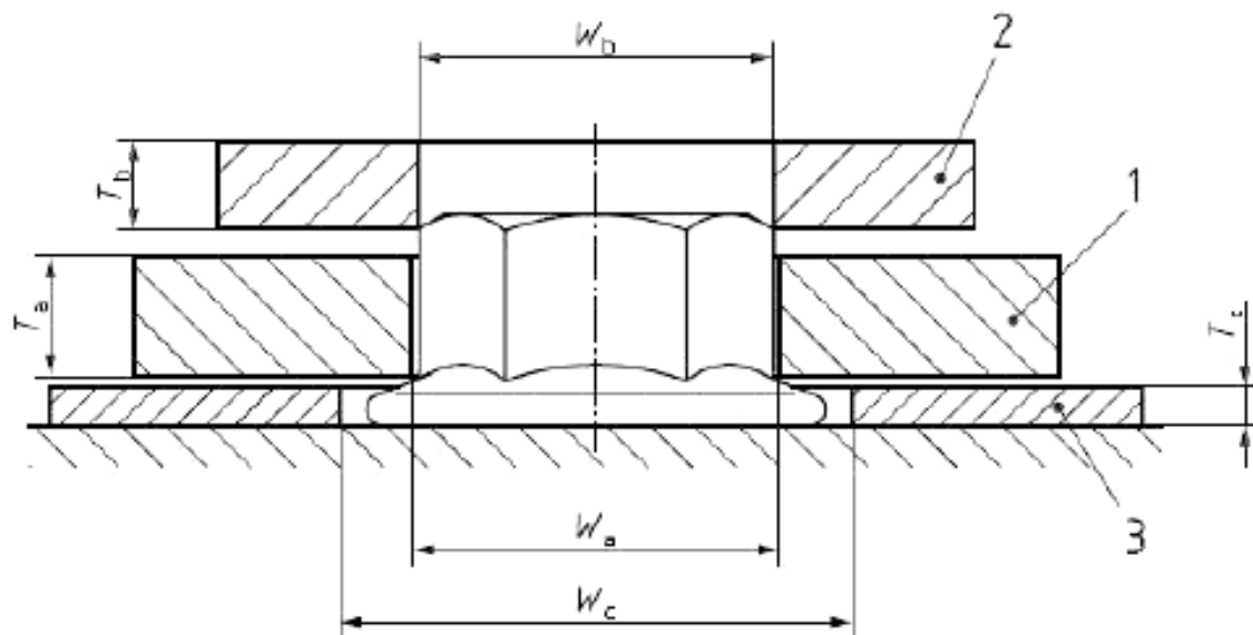
1 — калибр А; 2 — калибр В; 3 — калибр С; W_{a, \text{мин}} = e_{\text{теор}} ; W_{b, \text{макс}} = e_{\text{мин}} - 0,01 \text{ мм} ; T_{a, \text{макс}} = m_{\text{н}} \text{ мин}
