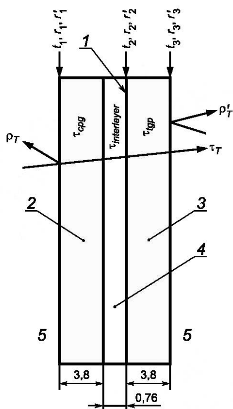
1 — поверхность с покрытием; 2 — лист бесцветного стекла (3,8 мм); 3 — лист окрашенного в массе стекла (3,8 мм); 4 — промежуточный слой (0,76 мм); 5 — воздух
