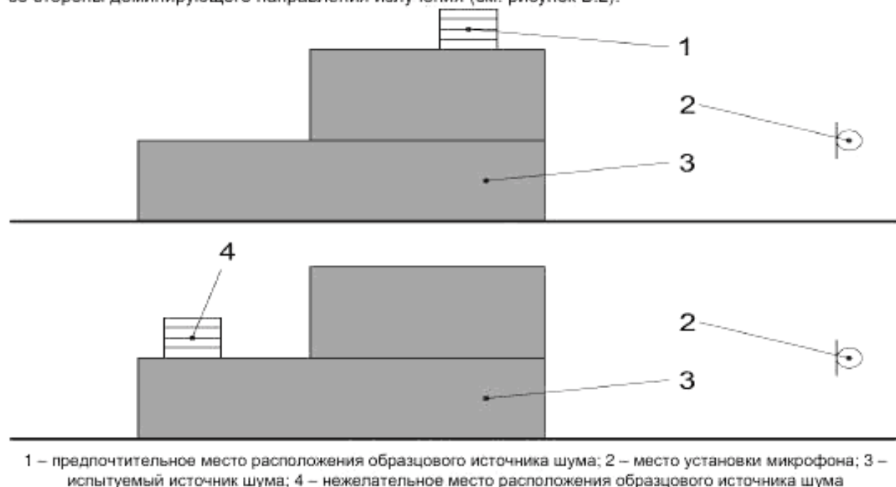
Рисунок В.1 – Места расположения образцового источника шума в случае испытуемого источника шума с ненаправленным излучением
