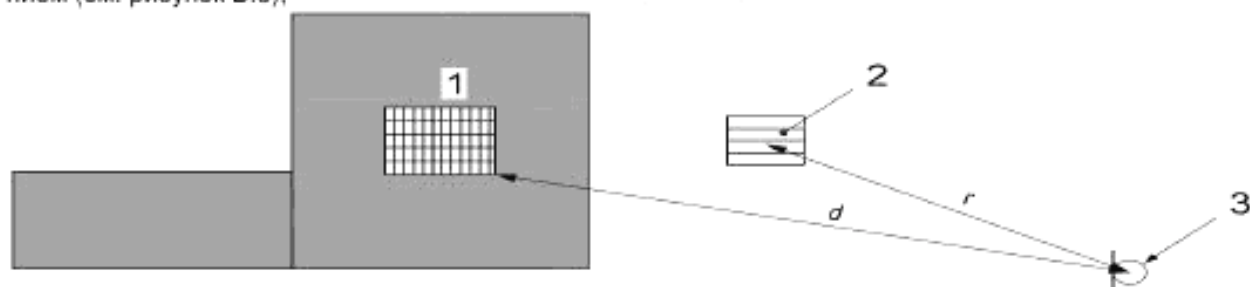
1 – элемент испытуемого источника шума с доминирующим излучением; 2 – место расположения образцового источника шума; 3 – место установки микрофона; d – расстояние от микрофона до элемента испытуемого источника с доминирующим излучением; r – расстояние от образцового источника шума до микрофона
