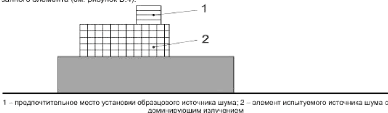
Рисунок В.3 – Место расположения образцового источника шума при наличии у испытуемого источника шума элемента с доминирующим ненаправленным излучением
