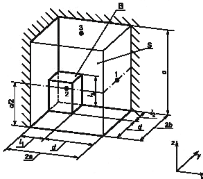
Рисунок С.7 — Измерительная поверхность в виде параллелепипеда с четырьмя точками установки микрофонов при испытаниях устанавливаемых на полу источников шума в случае двух звукоотражающих плоскостей
