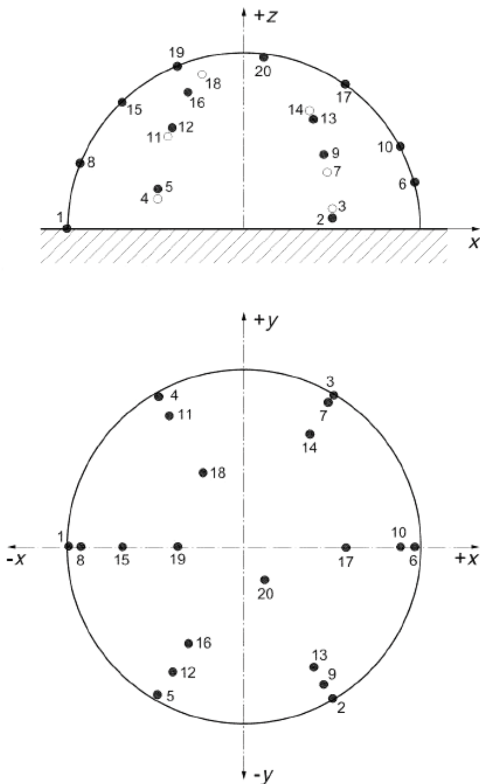
Рисунок Е.2 – Точки измерений на полусферической измерительной поверхности (случай источника широкополосного шума)
