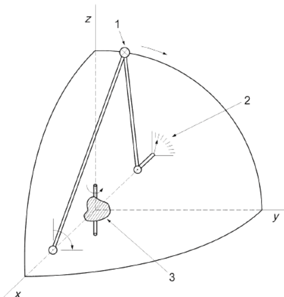
1 – микрофон; 2 – устройство отсчета зенитного угла (косинусный потенциометр); 3 – источник шума на поворотной платформе
