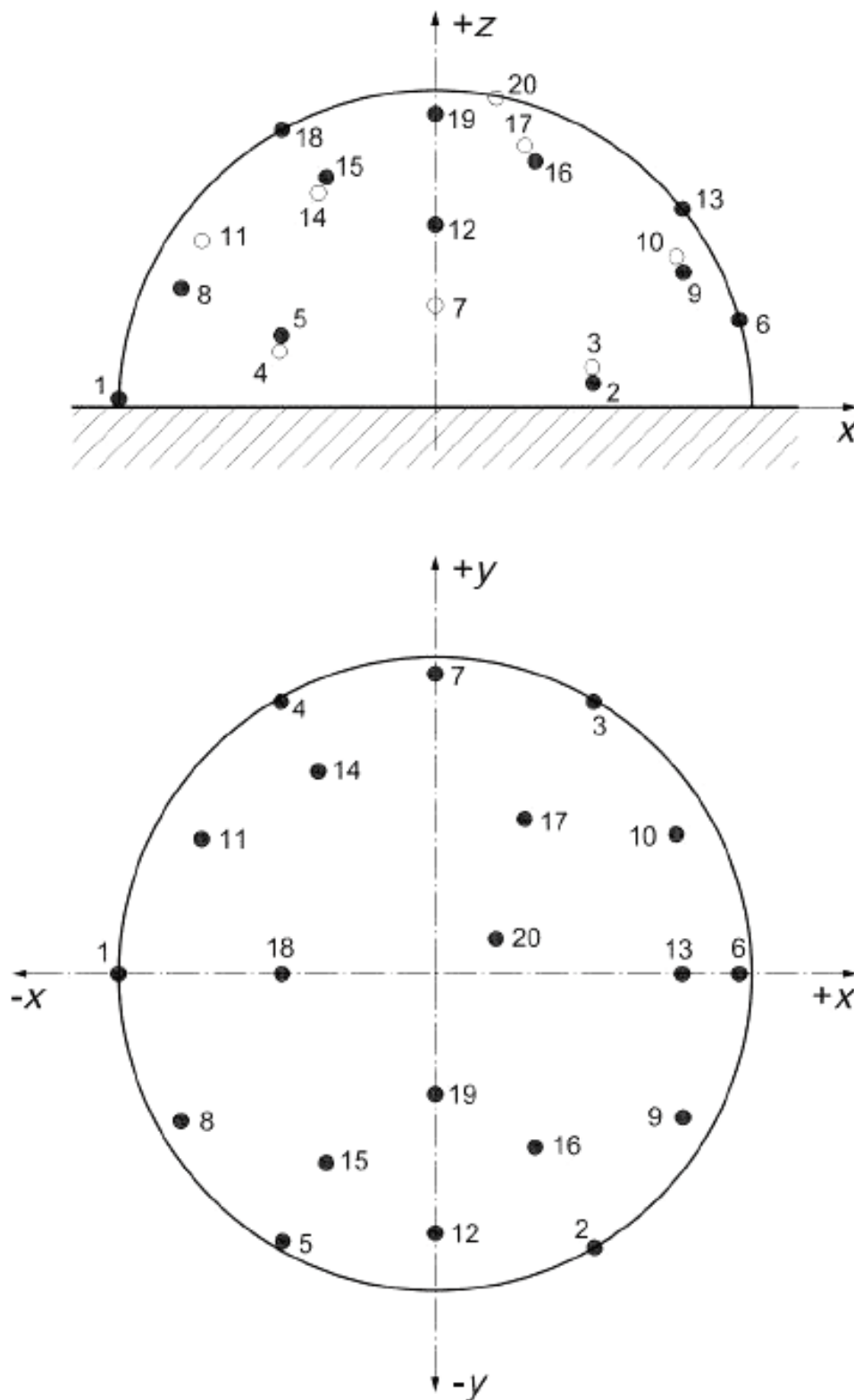
Рисунок Е.1 – Точки измерений на полусферической измерительной поверхности (общий случай)
