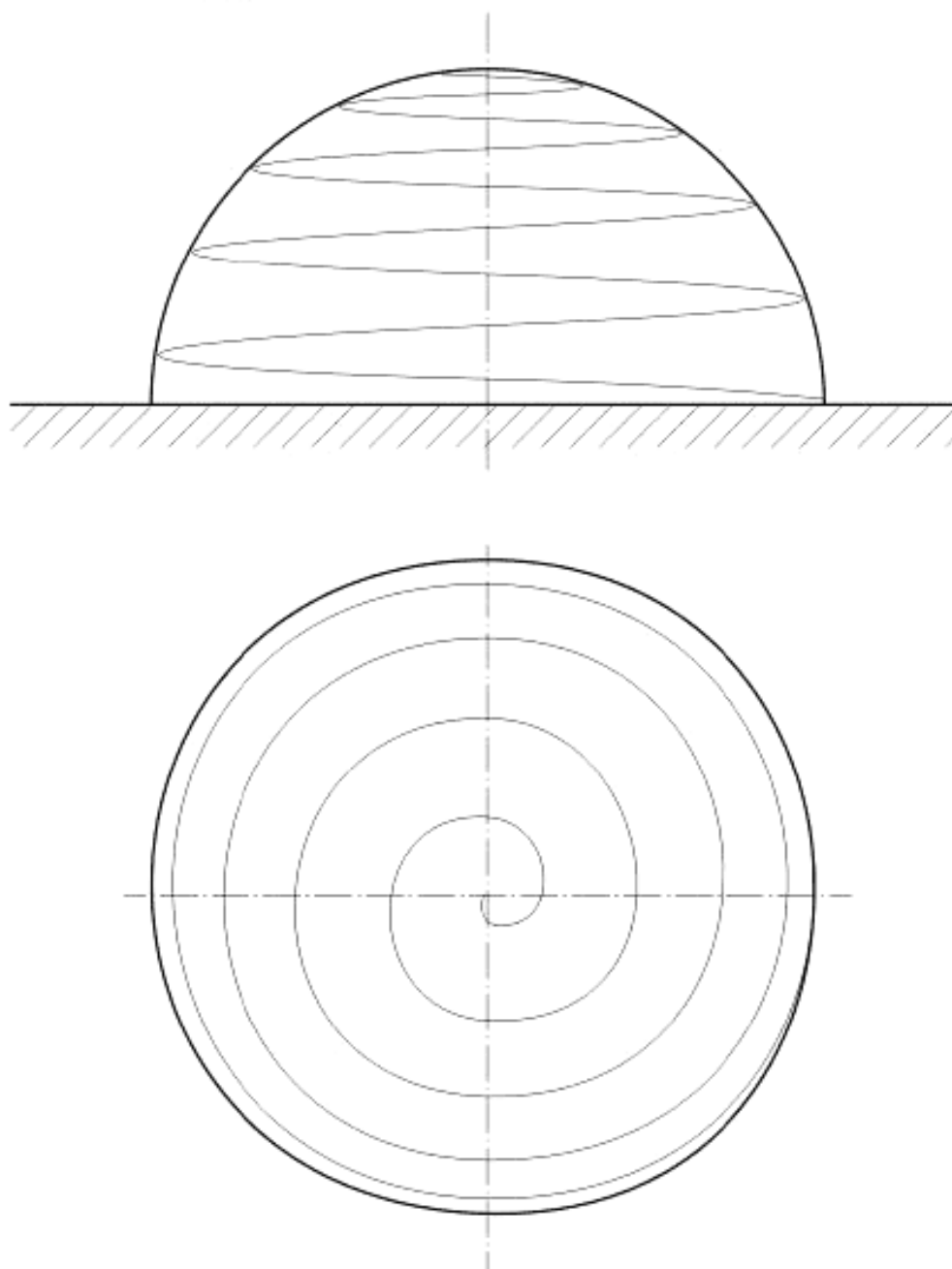
Рисунок Н.1 – Винтовая траектория перемещения микрофона по полусферической измерительной поверхности
