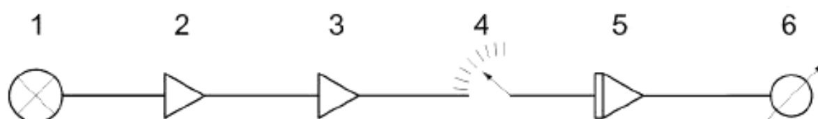
1 – микрофон; 2 – усилитель и анализатор спектра; 3 – квадратичный усилитель; 4 – косинусный потенциометр; 5 – интегратор; 6 – показывающее устройство
