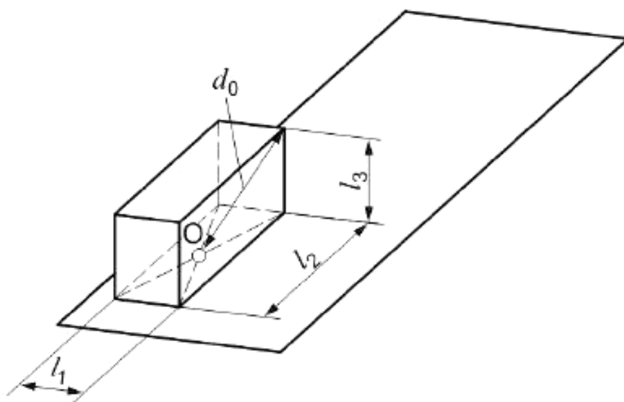
б) Заглушенная камера со звукоотражающим полом (полузаглушенная камера),
