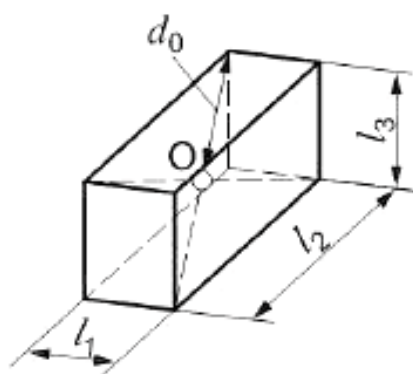
а) Заглушенная камера, d_0 = \sqrt{(l_1/2)^2 + (l_2/2)^2 + (l_3/2)^2}
