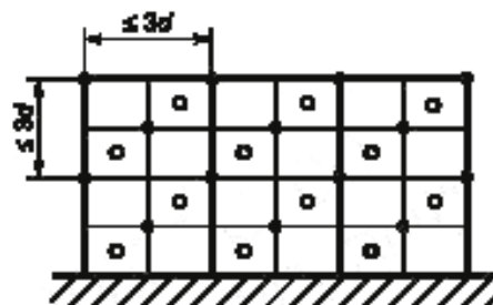
• — основные точки установки микрофонов; ○ — дополнительные точки установки микрофонов; d — измерительное расстояние
