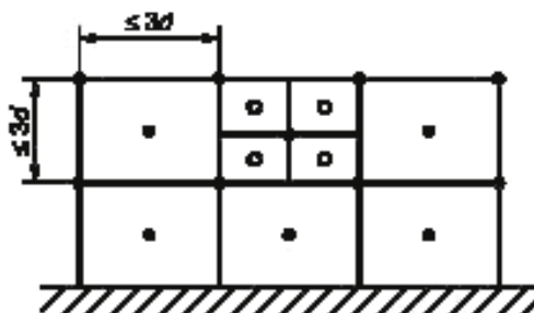
• — основные точки установки микрофонов; ○ — дополнительные точки установки микрофонов; d — измерительное расстояние
