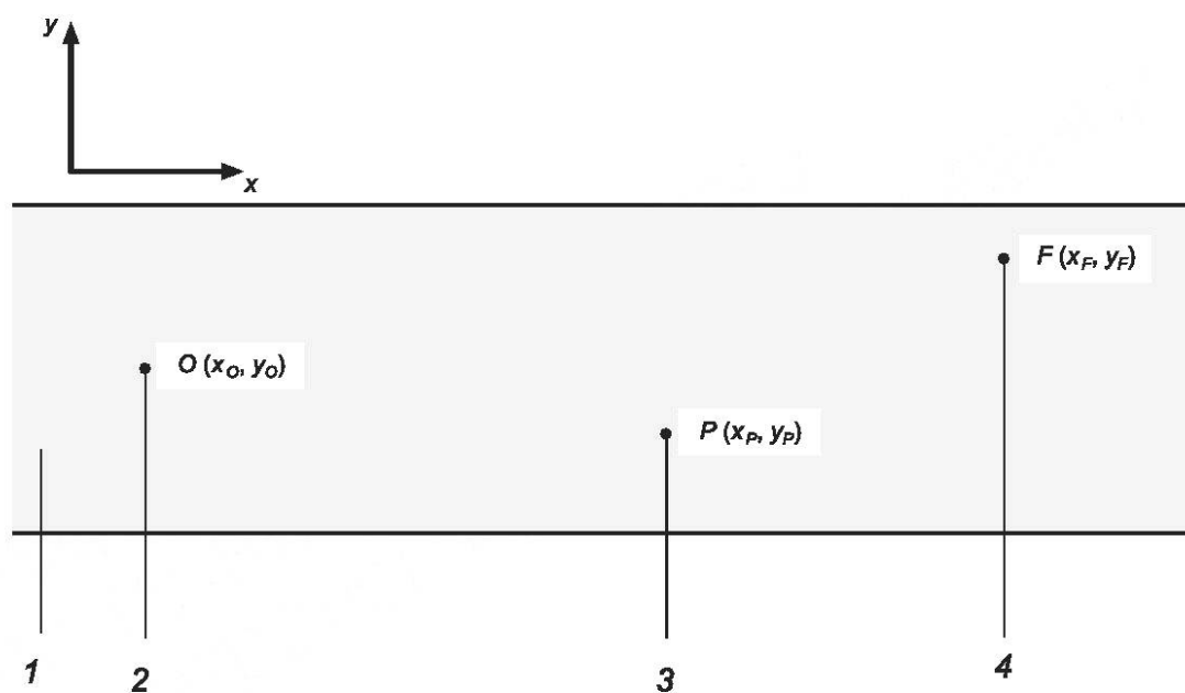
Рисунок 3 — Координаты точек расположения ОП, наблюдателя и расчетной точки на дороге (в плане)
