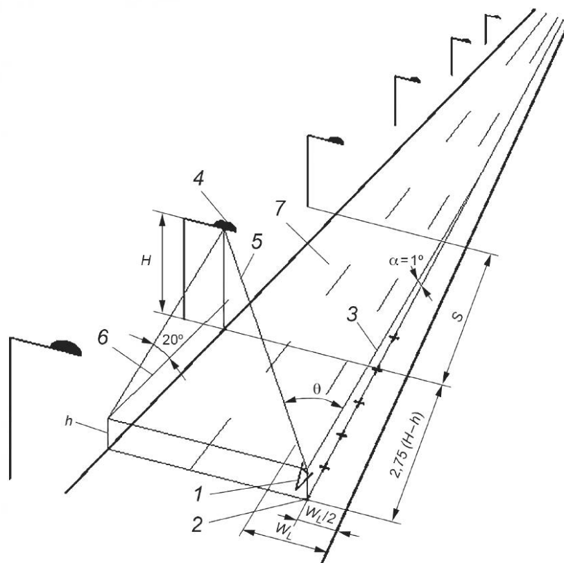
1 — глаз наблюдателя; 2 — точки расположения наблюдателя (помечены значком «+»); 3 — линия зрения; 4 — ОП; 5 — плоскость экранирования; 6 — линия горизонта; 7 — расчетное поле; S — шаг ОП; h — высота расположения глаза наблюдателя над дорогой; W_L — ширина полосы движения; H — высота светового центра ОП над дорогой; \theta — угол между линией зрения наблюдателя и направлением на ОП
