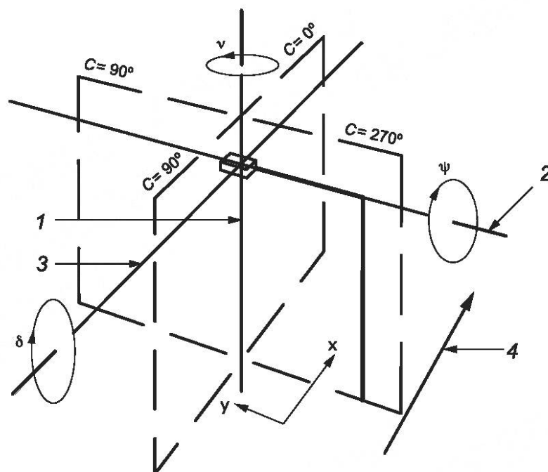
Рисунок 5 — Расположение главных осей ОП и положительные направления вращения системы координат ОП из положения при измерении в положение при использовании
