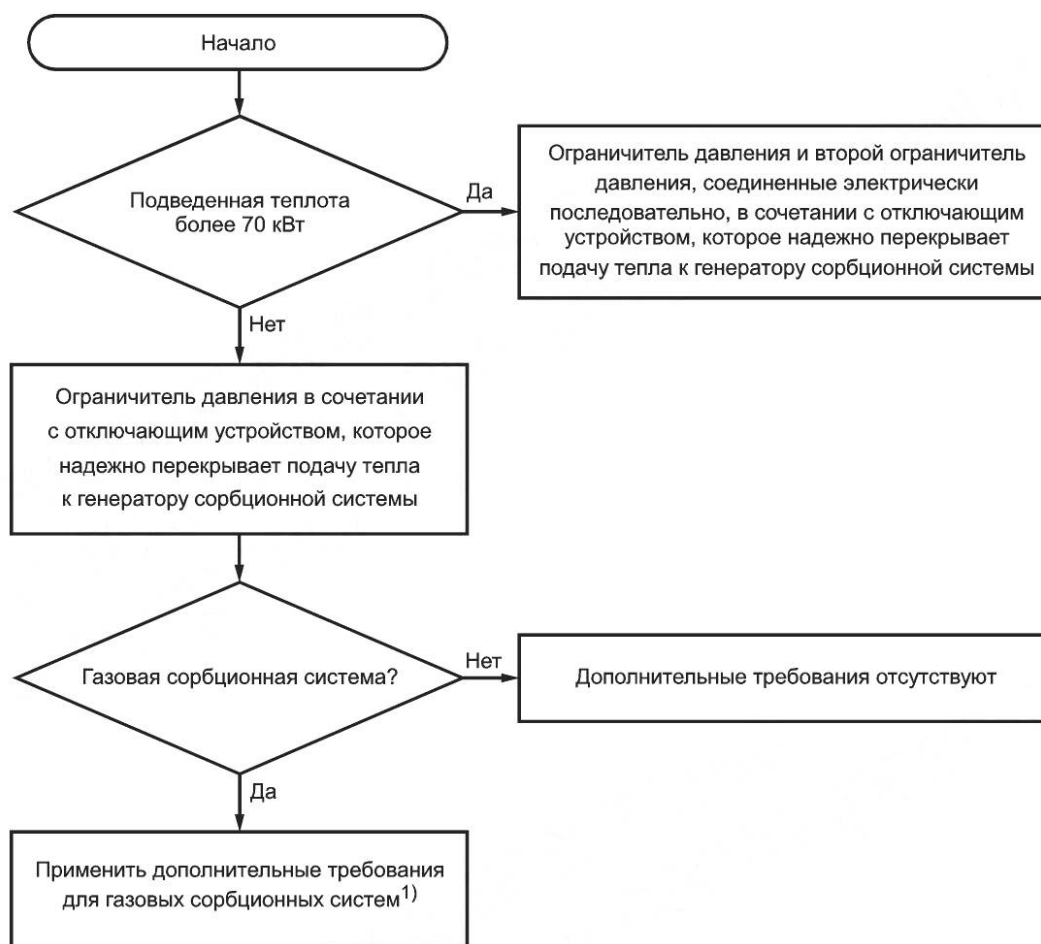
Рисунок 1 — Защита холодильной системы от избыточного давления
