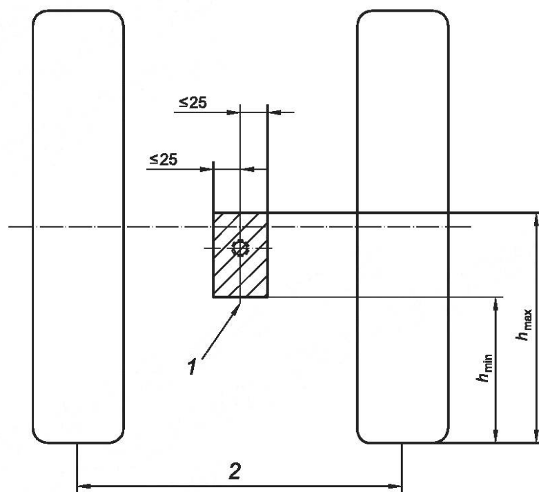
Рисунок 1 — Расположение переднего ВОМ (вид спереди трактора)
