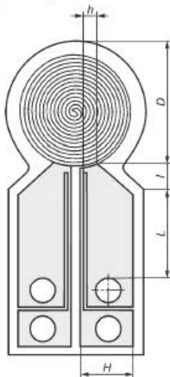
Рисунок 2 — Датчик с нагретым диском с бифилярной спиралью в качестве нагревательного/чувствительного элемента
