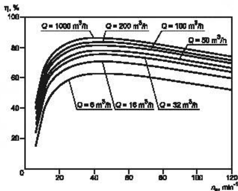
Рисунок 3 — Зависимости КПД от n_d , полученные для консольного насоса (тип К) с частотой вращения вала n_N = 2900 \text{ мин}^{-1} , MEI = 0,7 и различными значениями Q_{BEP}
