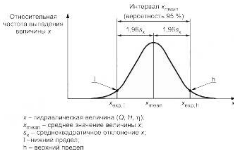
Рисунок С.1 — Нормальное распределение величины типоразмера насоса
