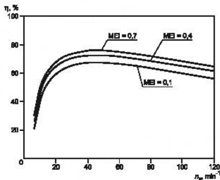
Рисунок 4 — Зависимости КПД от n_d , полученные для консольного насоса (тип К) с частотой вращения вала n_N = 2900 \text{ мин}^{-1} , подачей Q_{BEP} = 32 \text{ м}^3/\text{ч} и различными значениями MEI
