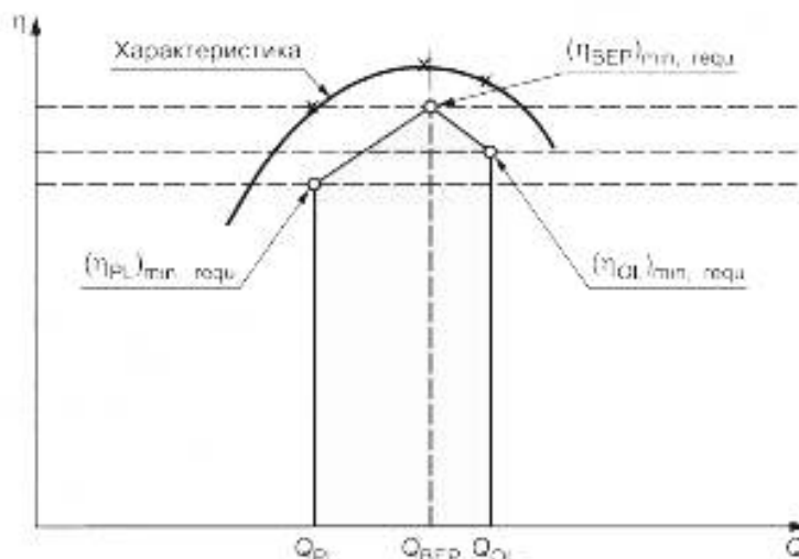
Рисунок 2 — Концепция определения энергоэффективности
