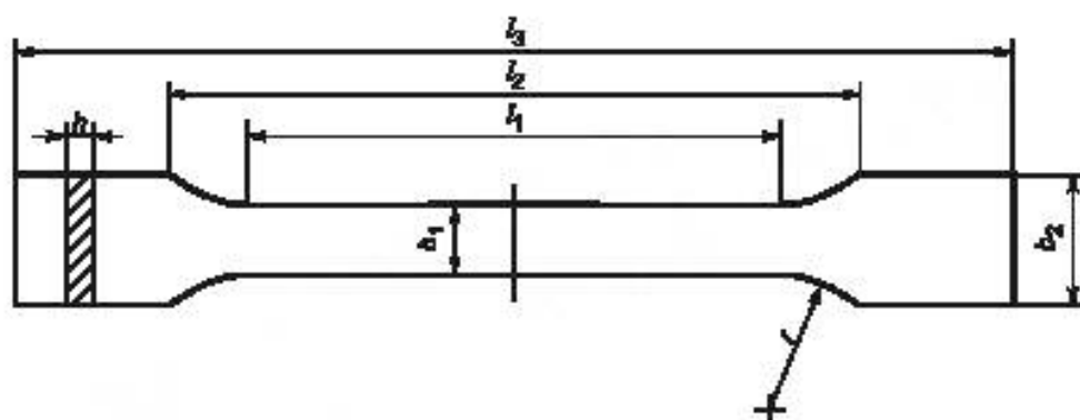
Рисунок 1 — Типовой образец для испытания на растяжение
