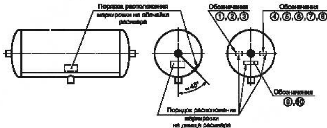
Рисунок 3 — Расположение маркировки, наносимой на стенку ресивера
