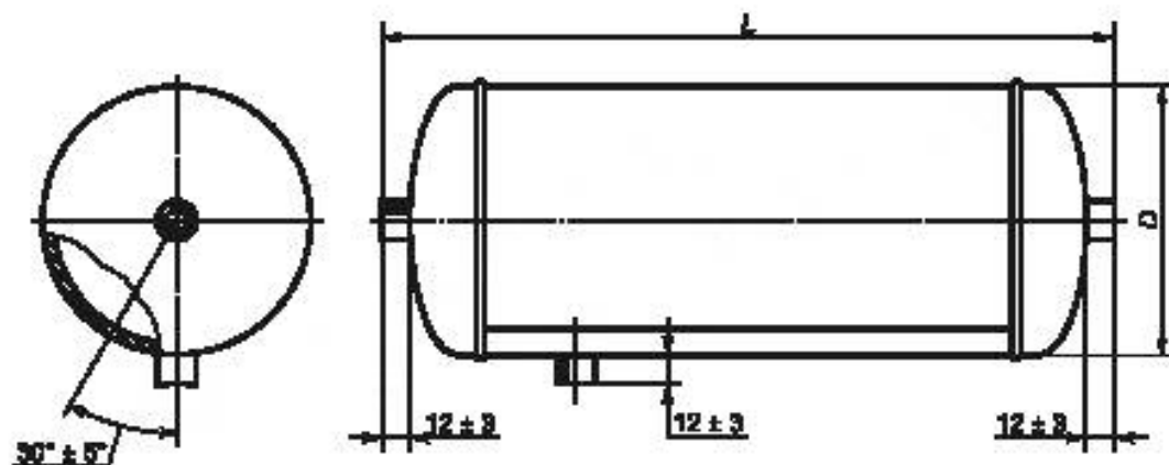
Рисунок 1 — Ресивер Тип 1
