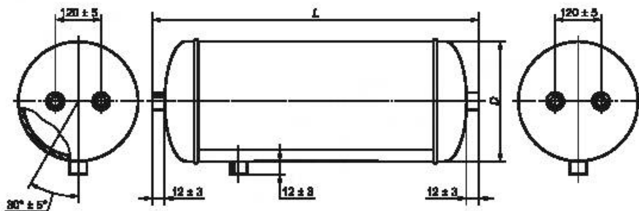
Рисунок 2 — Ресивер Тип 2
