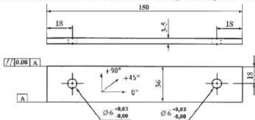
Рисунок 3 — Образец ПК с двумя отверстиями
