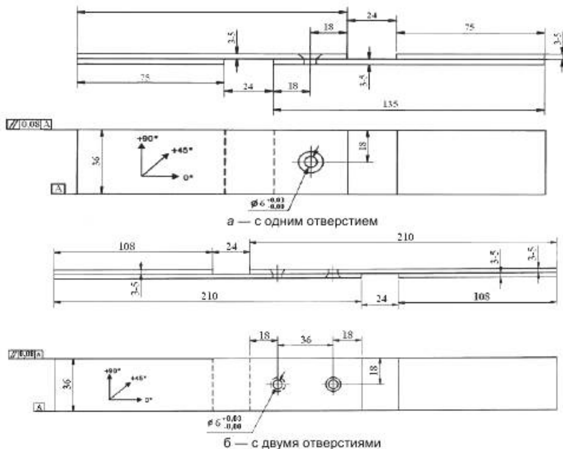
Рисунок 4 — Составной образец ПК
