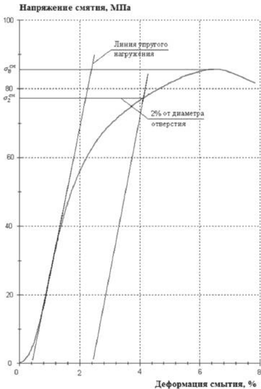
Рисунок 6 — Диаграмма смятия
