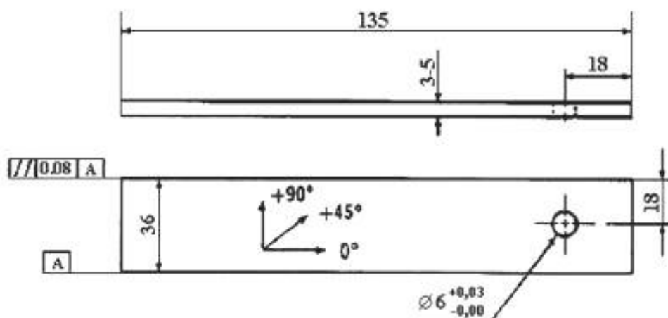
Рисунок 2 — Образец ПК с одним отверстием
