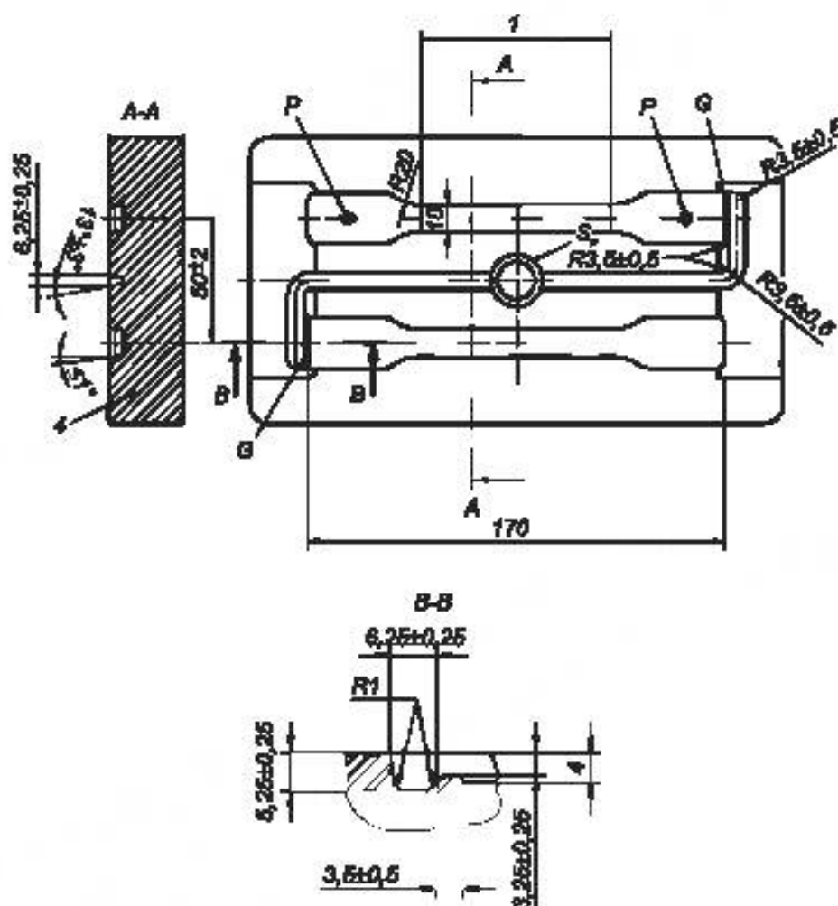
T – предпочтительно 82 мм; S_p – вертикальный литник; G – литник; P – датчик давления (не является обязательным элементом) Рисунок 2 – Форма ИСО типа А с двумя полостями
