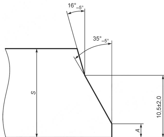
A — ширина торцевого притупления, S — толщина стенки
