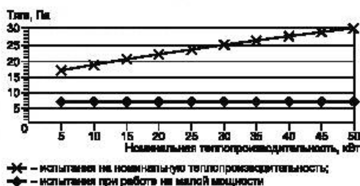
Рисунок 2 — Значения тяги в дымоходе
