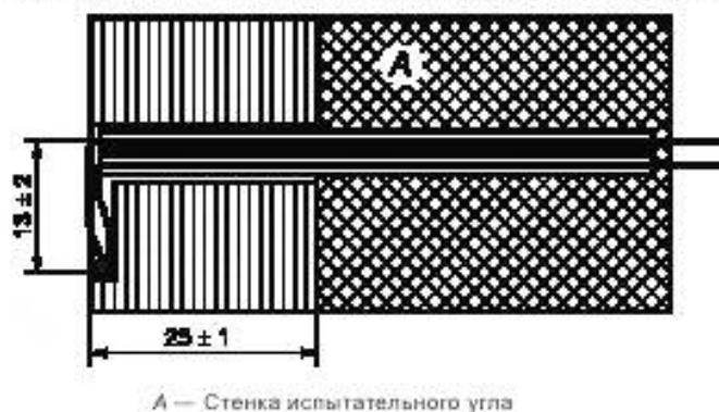
Рисунок А.7 — Расположение термоэлемента в стенке испытательного угла
