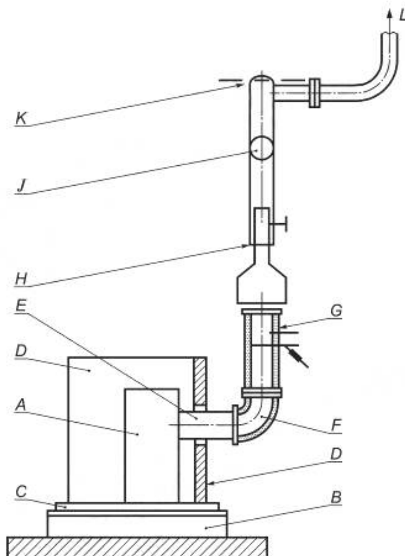
А — котел; В — платформенные весы контроля выгорания топлива; С — пол испытательного угла; D — боковая стенка испытательного угла; E — дымоход; F — переходник для дымовых газов (колени); G — измерительный участок; H — регулируемая часть трубы; J — регулируемая дроссельная заслонка; K — вентилятор; L — выпуск в атмосферу
