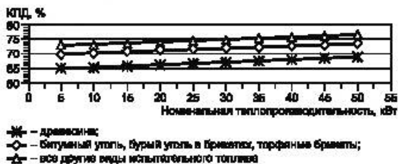
Рисунок 1 — КПД при номинальной теплопроизводительности
