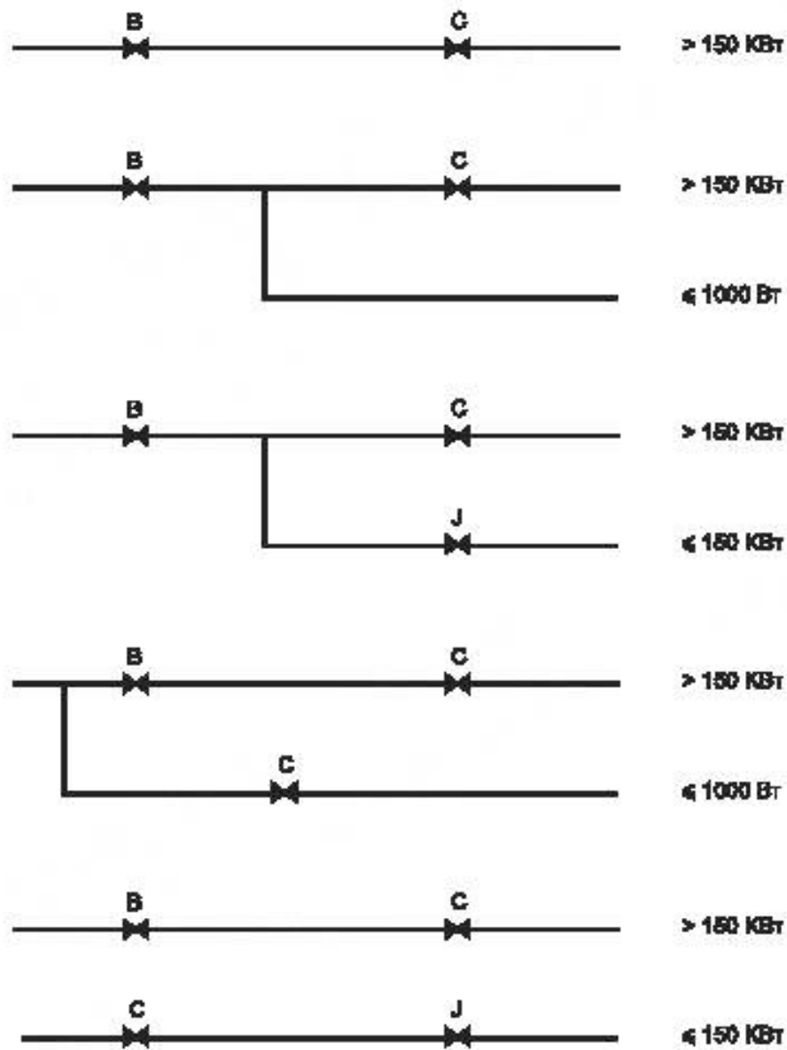
Рисунок Н.2 — Подводимая тепловая мощность до 300 кВт
