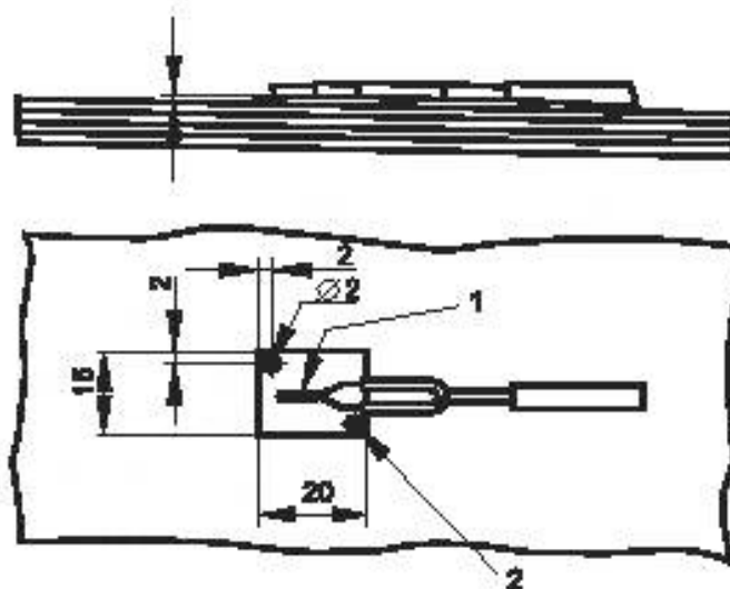
Рисунок 13 — Крепление термопары к испытательной панели для измерения температуры пола под котлом
