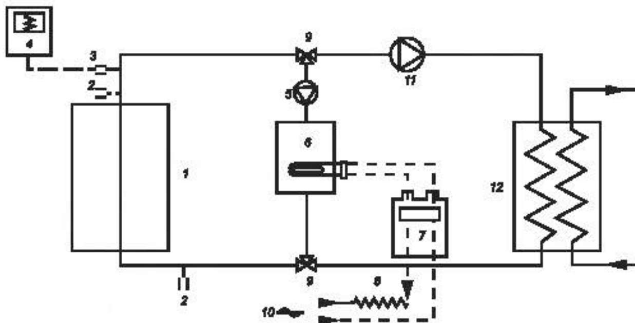
1 – испытуемый котел; 2 – датчик температуры; 3 – низкоинерционный термозлемент; 4 – записывающее устройство; 5 – насос (обеспечивает перепад температур между обоими термодатчиками в пределах 2 °С – 4 °С от максимальной испытательной температуры); 6 – электрический водонагреватель; 7 – электросчетчик; 8 – регулятор напряжения; 9 – клапан на 1/4 лаворота; 10 – электропитание; 11 – вспомогательный насос (при необходимости); 12 – теплообменник
