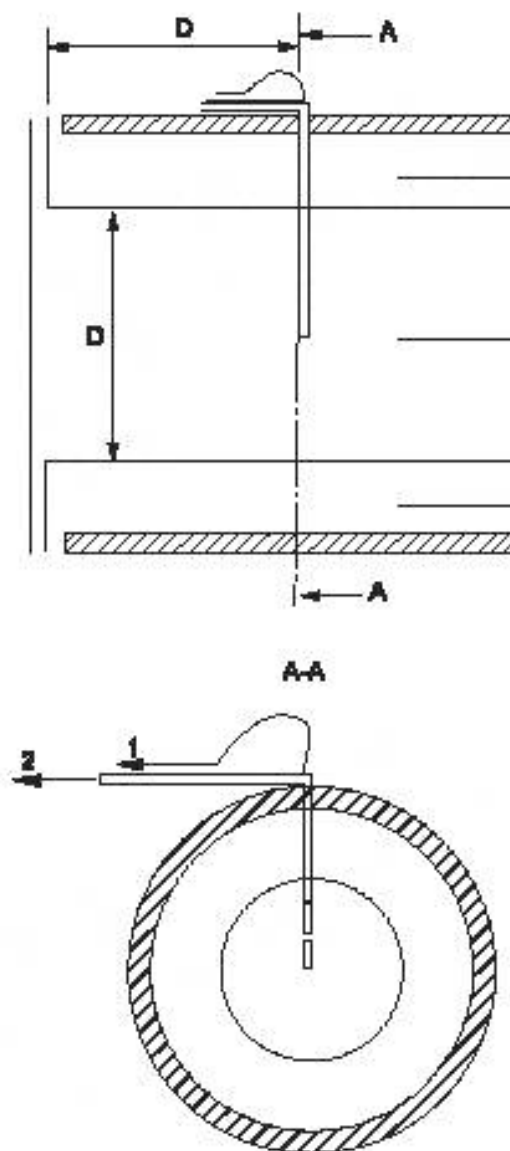
Рисунок 4 — Положение зонда пробоотборника для котлов типа С
