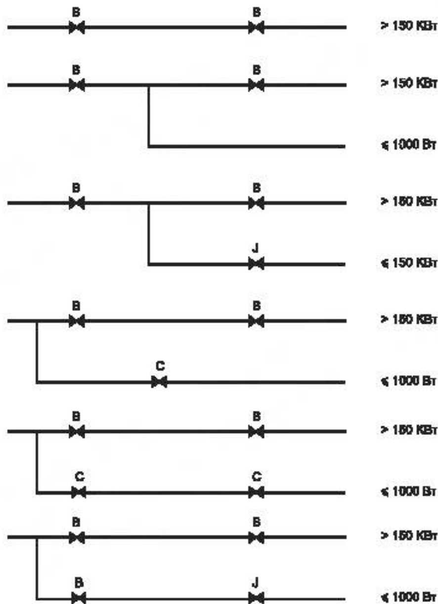
Рисунок Н.4 — Подводимая тепловая мощность до 300 кВт
