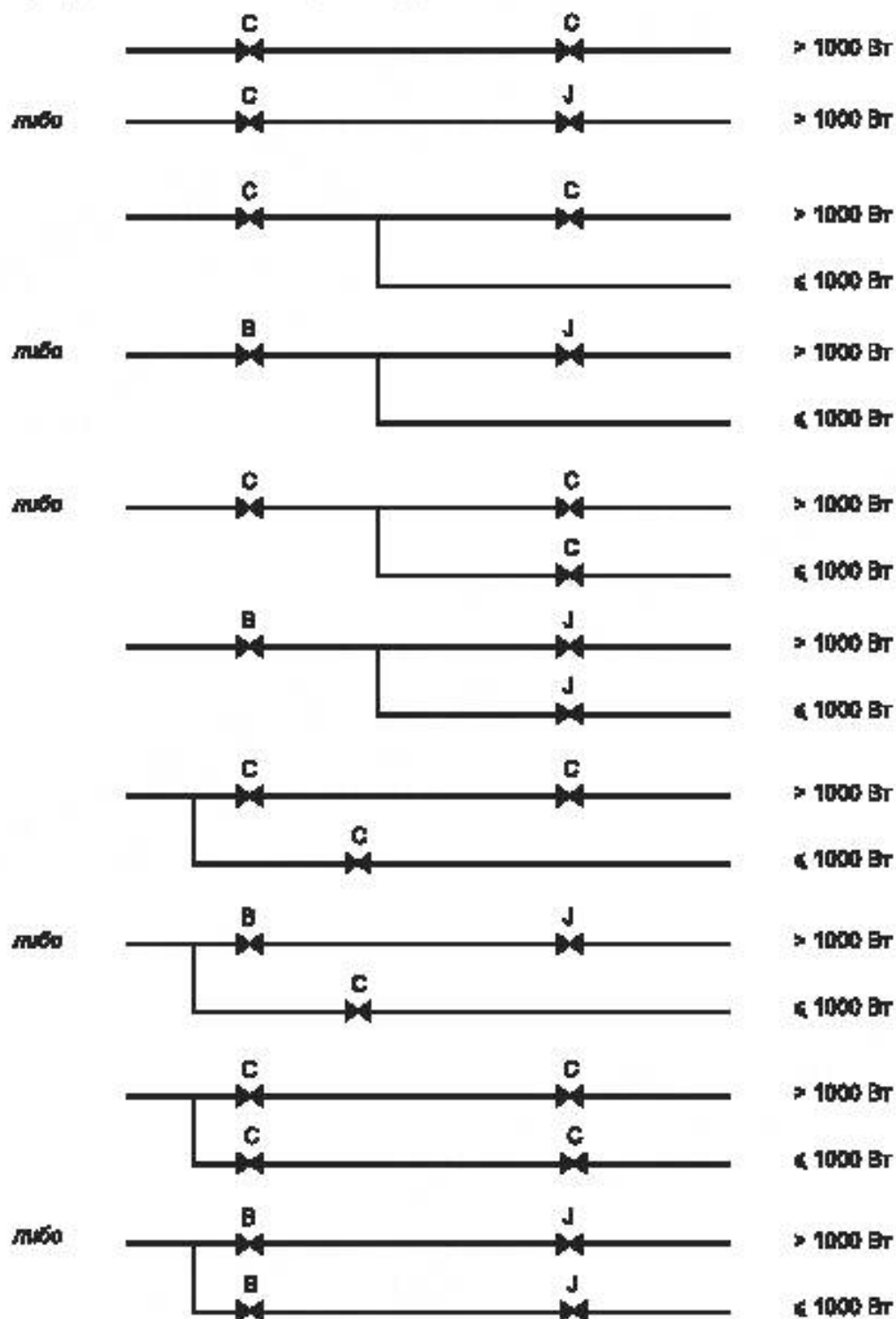
Рисунок Н.3 — Подводимая тепловая мощность до 150 кВт
