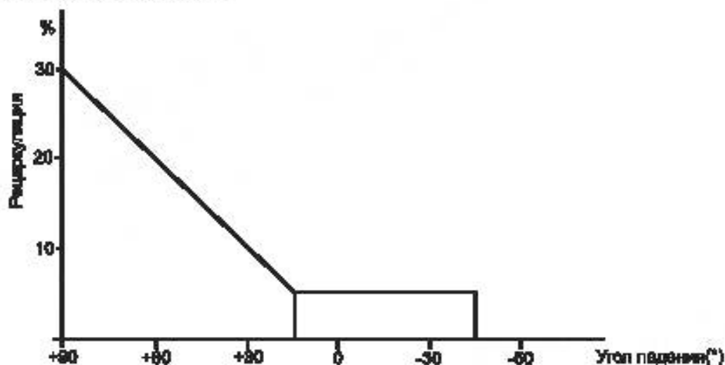
Рисунок N.1 – Максимальная допустимая рециркуляция продуктов сгорания
