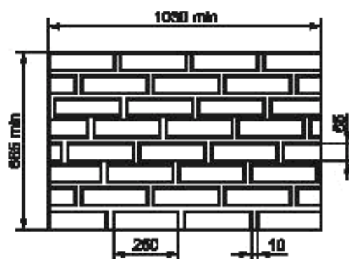
Рисунок 2 — Экран «кирпичная стена»
