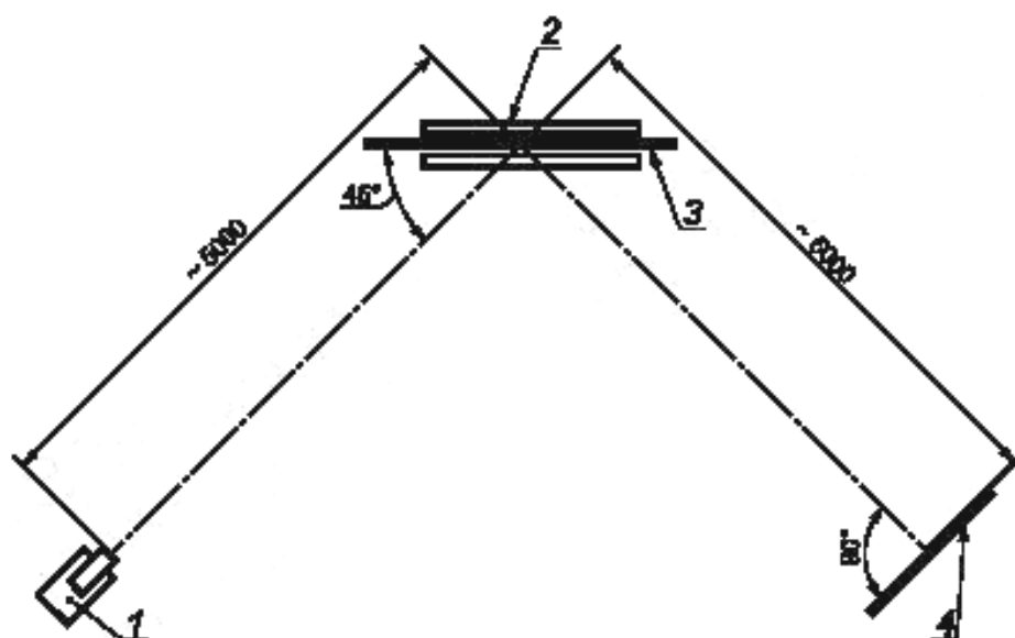
1 — диалпроектор с растром; 2 — держатель образцов; 3 — образец стекла; 4 — экран
