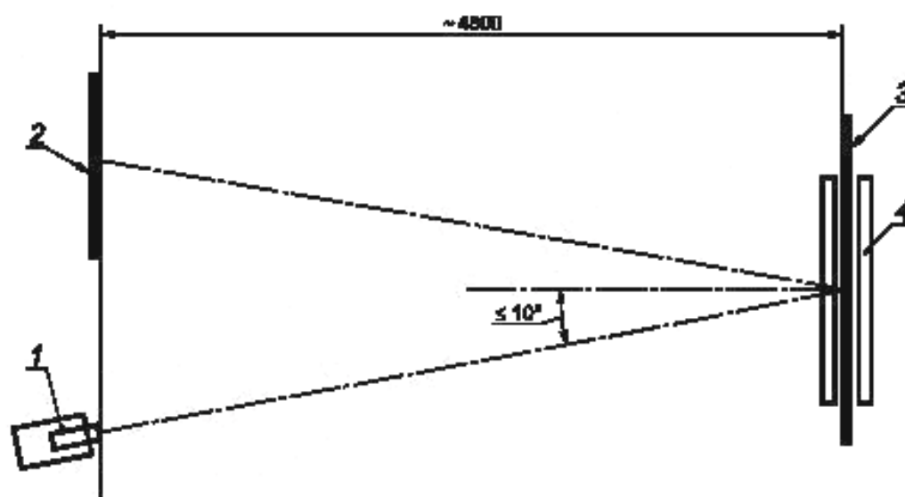
Рисунок 4 — Определение оптических искажений в отраженном свете (метод А)
