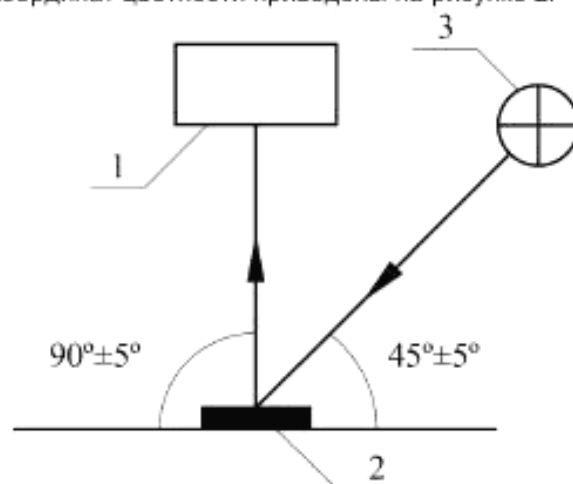
Рисунок 2 – Условия измерения координат цветности и коэффициента яркости
