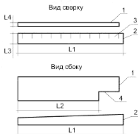
1 – планка; 2 – клин; 3 – измерительная шкала; 4 – паз планки; L1 – длина основания клина; L2 – длина основания планки; L3 – ширина основания клина; L4 – ширина основания планки
