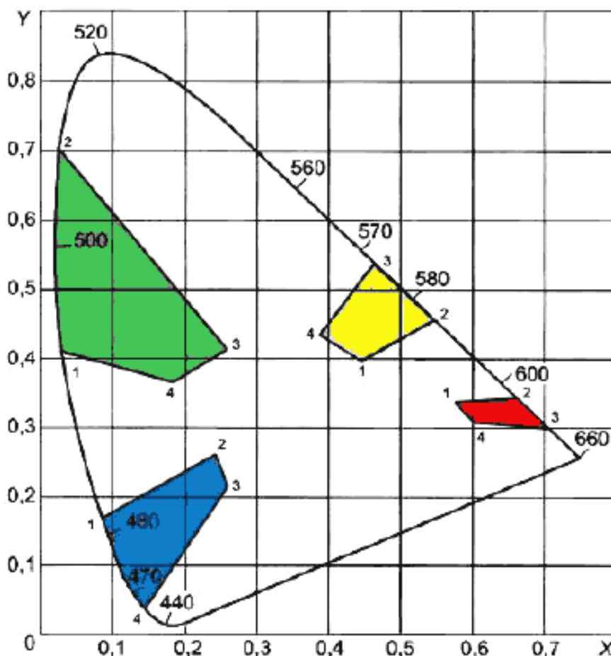
Рисунок 1 — График цветных областей для ЦПП (МКО, 1931 г. [1])
