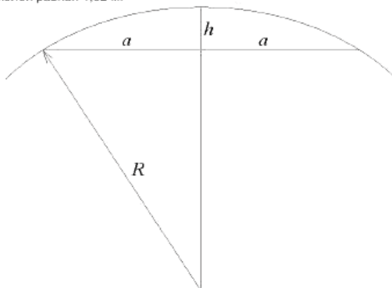
Рисунок 1 – Схема измерения радиуса кривой
