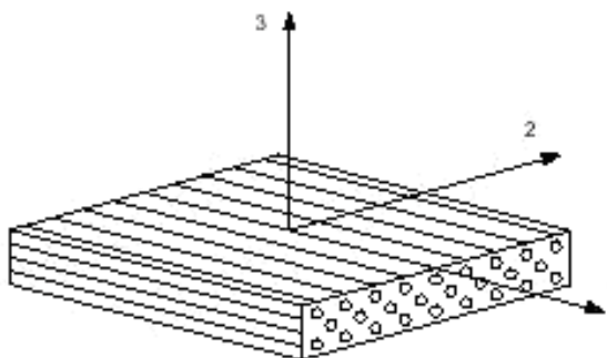
Рисунок 1 – Оси симметрии полимерного композита, армированного волокнами
