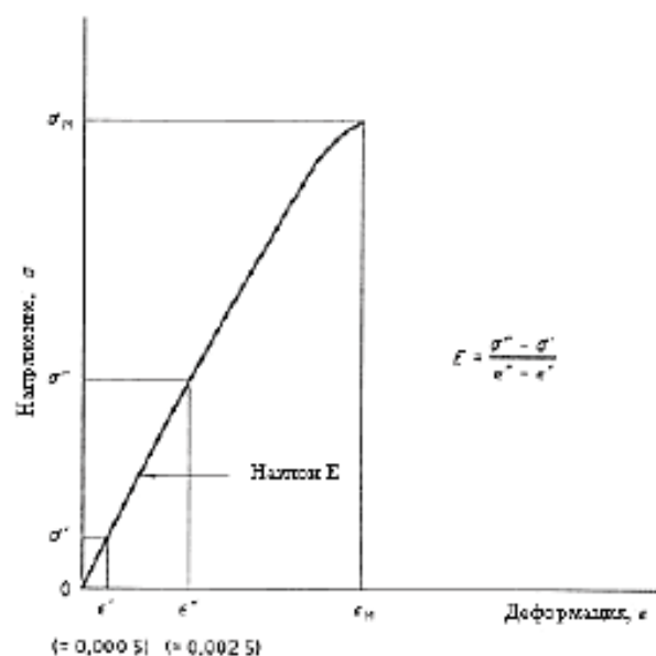
Рисунок 2 – Диаграмма напряжение-деформация
