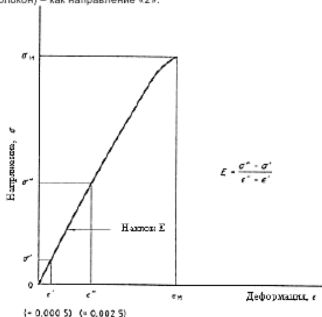
Рисунок 1 — Кривая напряжение — деформация
