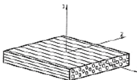
Рисунок 2 — Оси симметрии пластического композиционного материала, армированного волокнами
