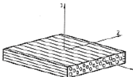
Рисунок 2 – Оси симметрии пластического композиционного материала, армированного волокнами
