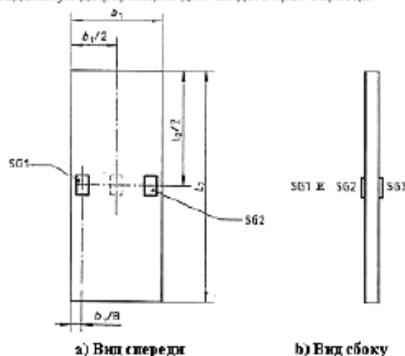
Рисунок В.1 —Размещение тензодатчиков (SG1, SG2 и SG3) для проверки центрирования системы
