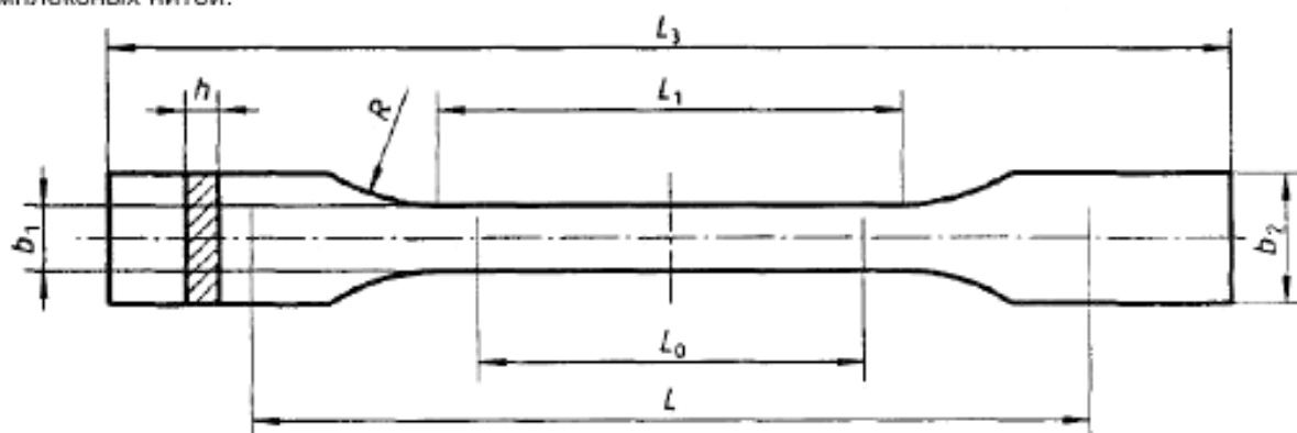
Рисунок 4 – Образец типа 1В
