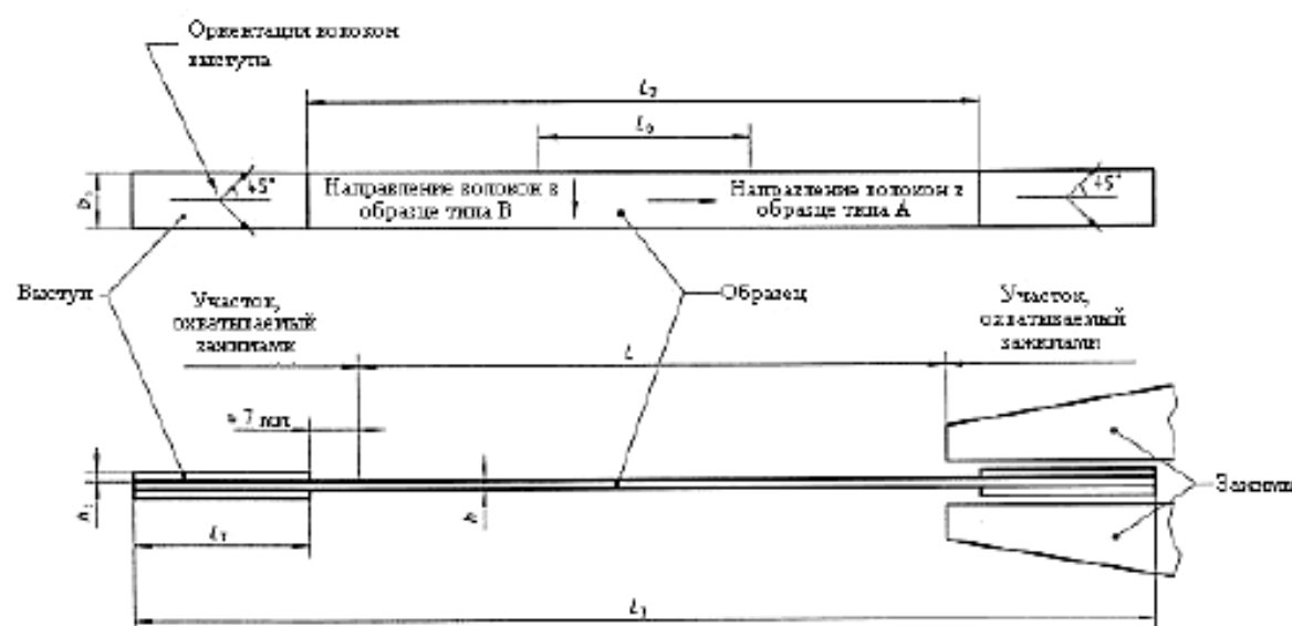
Рисунок 7 – Образцы типов А и В
