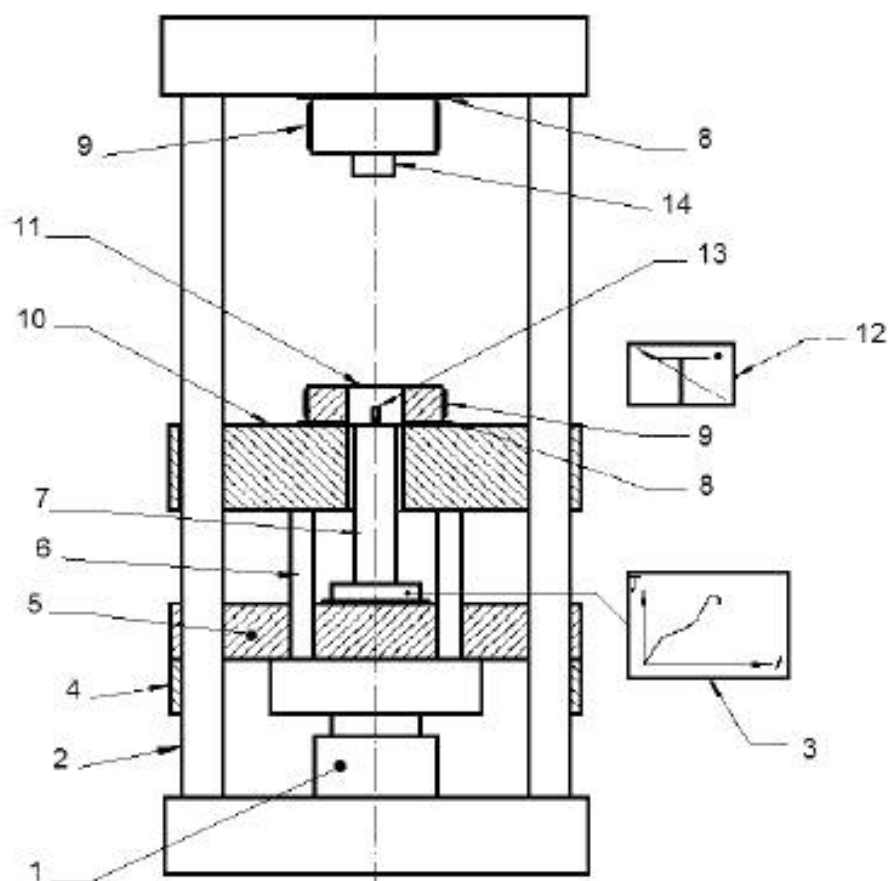
1 – управляемый давлением цилиндр, 2 – направляющие стойки, 3 – записывающее устройство температуры термозлемента, 4 - ограничитель, 5 - пластина выталкивателя, 6 - соединения стержней, 7 – выталкиватель, 8 – изоляционный щит, 9 – нагревательный элемент, 10 – поддержка формы, 11 – полость формы, 12 – контроль температуры формы, 13 – термозлемент, 14 – нагретый стальной пуансон.
