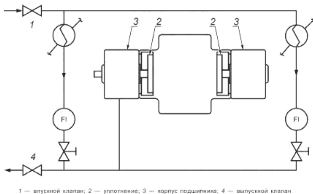
Рисунок Б.7 — Трубопровод для двухпорных насосов — Схема М, охлаждение теплообменников системы уплотнений
