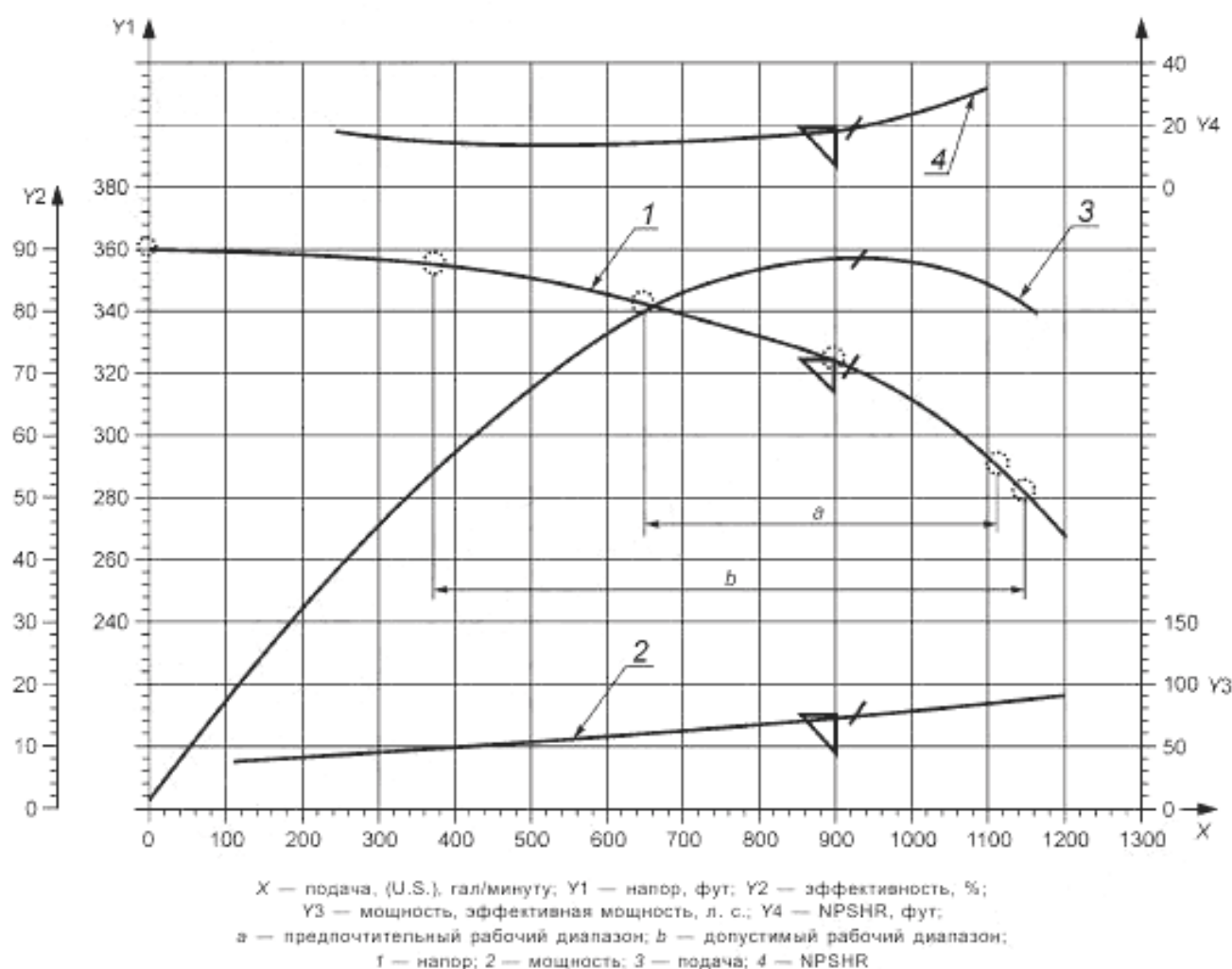
Рисунок П.3 — Форма представления испытательной кривой (единицы USC)
