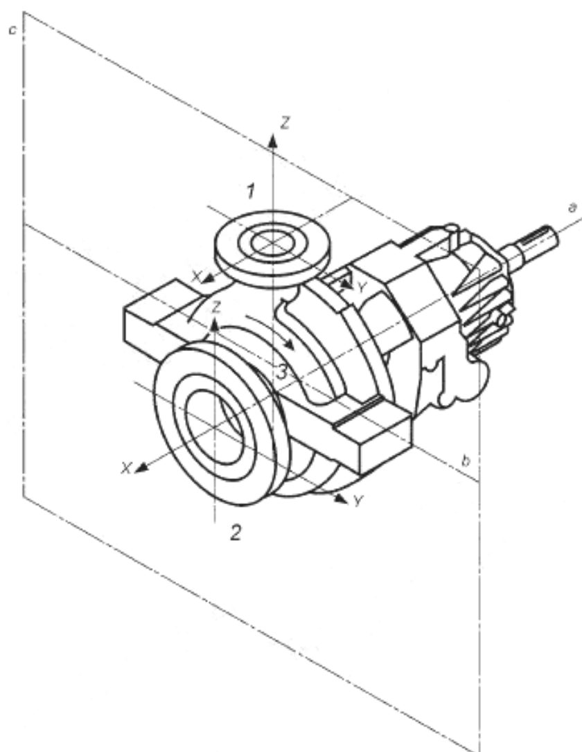
1 — нагнетательный патрубок; 2 — всасывающий патрубок; 3 — центр насоса; a — ось вала; b — ось основания; c — вертикальная плоскость
