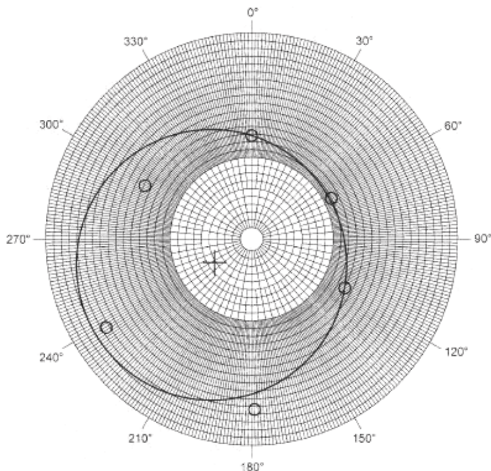
Рисунок Л.4 — Бланк для определения остаточного дисбаланса. Полярная диаграмма. Оптимально подобранная окружность для определения остаточного дисбаланса
