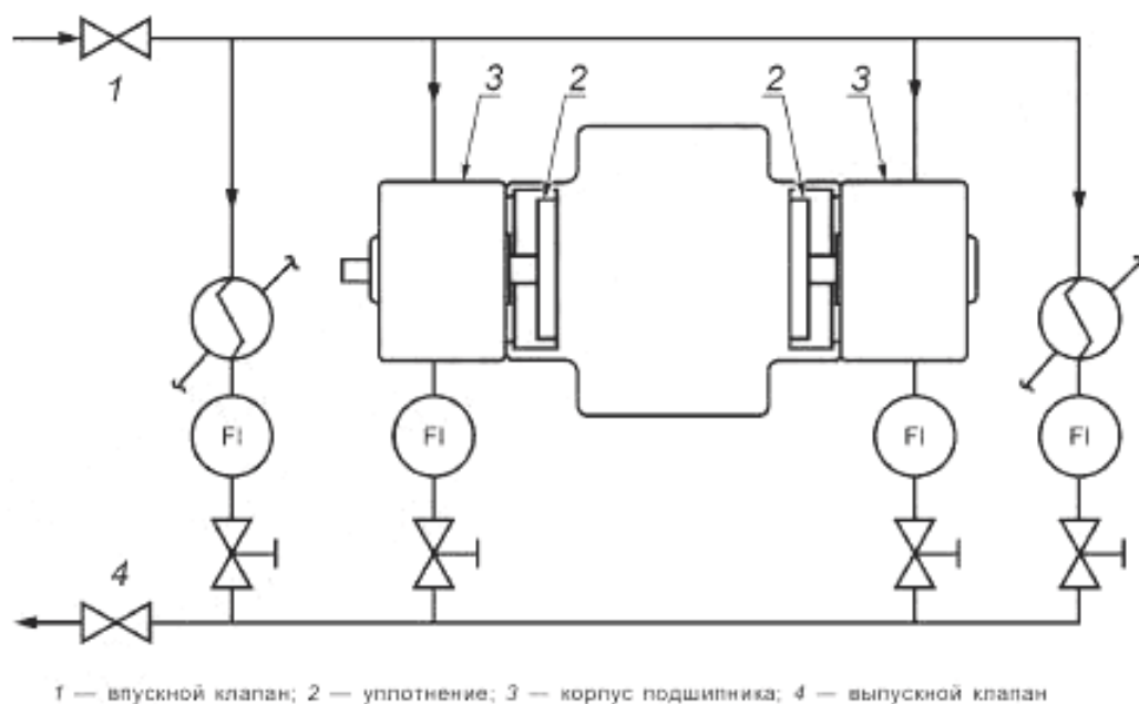
Рисунок Б.6 — Трубопровод для двухпорных насосов — Схема К, охлаждение подшипников параллельным потоком, идущим в теплообменник системы уплотнений
