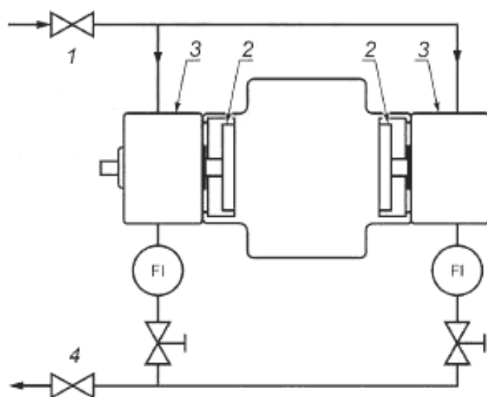
1 — впускной клапан; 2 — уплотнение; 3 — корпус подшипника; 4 — выпускной клапан
