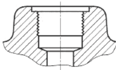
Рисунок 19 — Механически обработанная поверхность, пригодная для укладки и удержания прокладки при использовании цилиндрической резьбы
