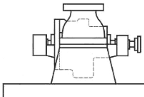
Рисунок 8 — Насос типа ВВ2
