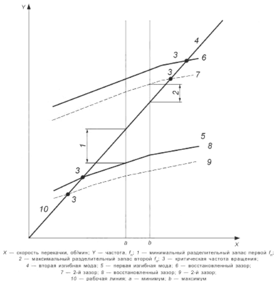
Рисунок К.2 — Типичная диаграмма Кэмпбелла
