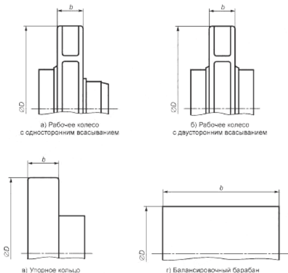
Рисунок 35 — Размеры вращающихся деталей, необходимые для балансировки в одной плоскости
