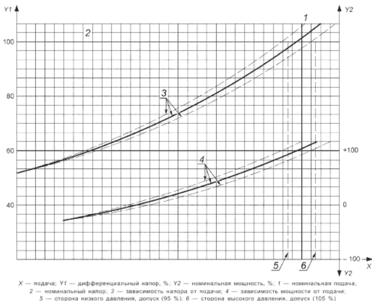
Рисунок В.2 — Испытательные допуски на параметры HPRT
