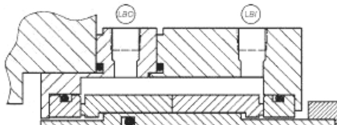
б) Компоновка «спиной к спине», 3CW-BB, контактное жидкостное уплотнение
