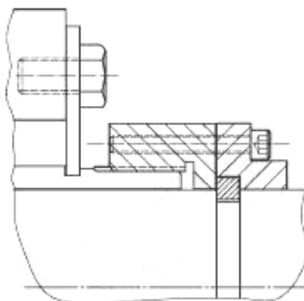
Рисунок 20 — Крепление втулки уплотнения разрезным кольцом
