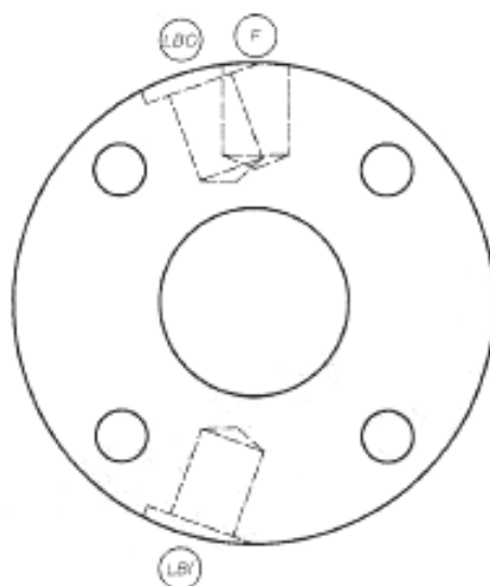
г) Типовая ориентация соединения фланца корпуса
