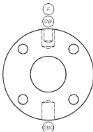
г) Типовая ориентация соединения фланца корпуса
