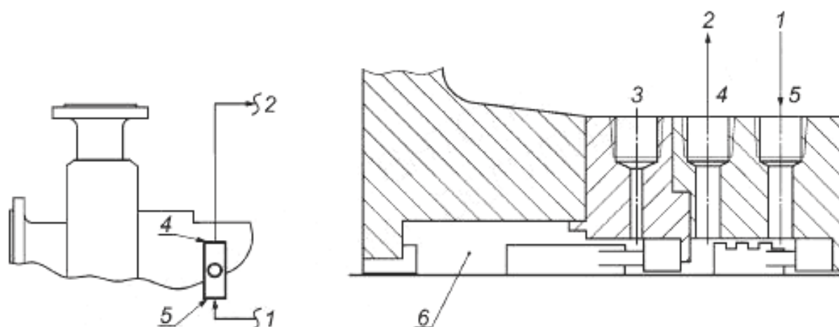
а) Трубопровод и схема измерительного прибора
