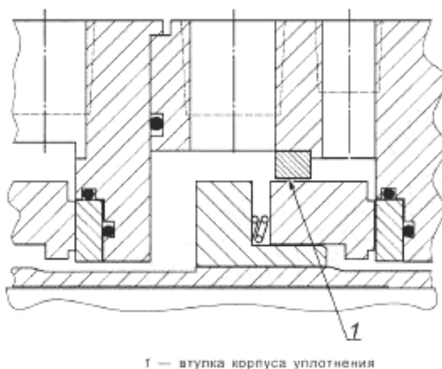
Рисунок 26 — Разрез втулки, находящейся в корпусе уплотнения, конфигураций 2CW-CS и 2NC-CS
