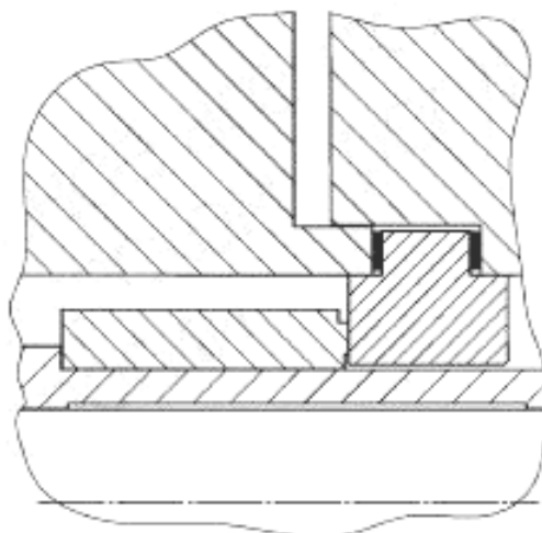
Рисунок 21 — Фиксация поверхностей
