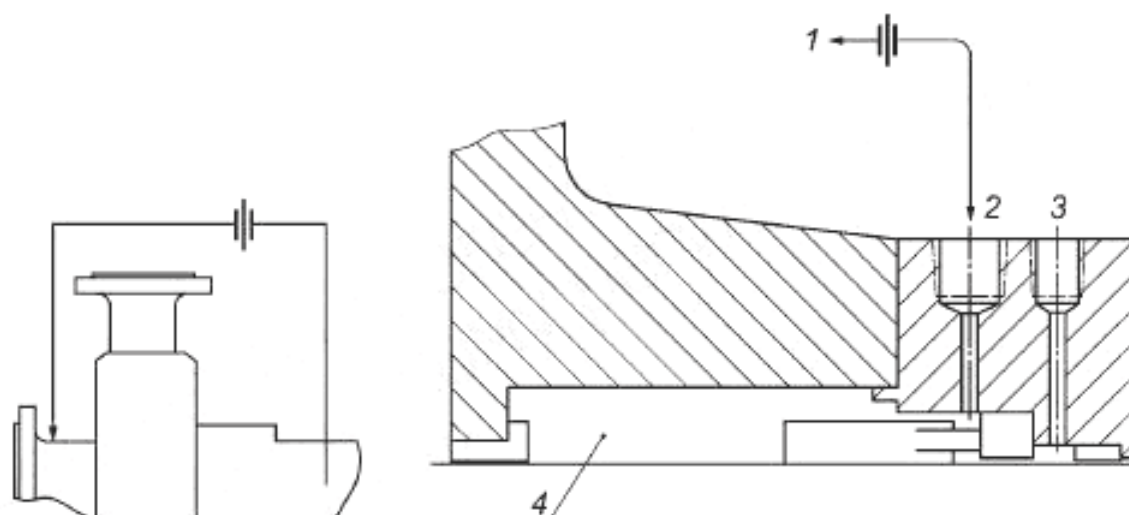
а) Трубопровод и схема измерительного прибора
