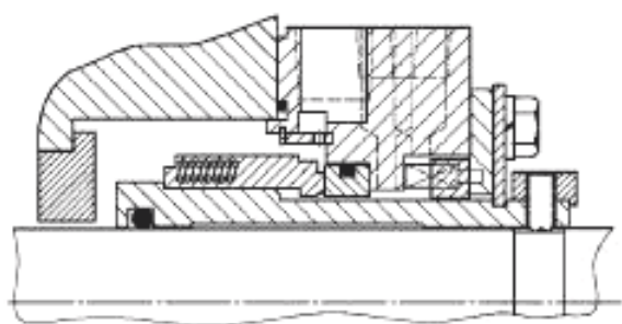
а) Стандартное (вращающийся упругий элемент)
