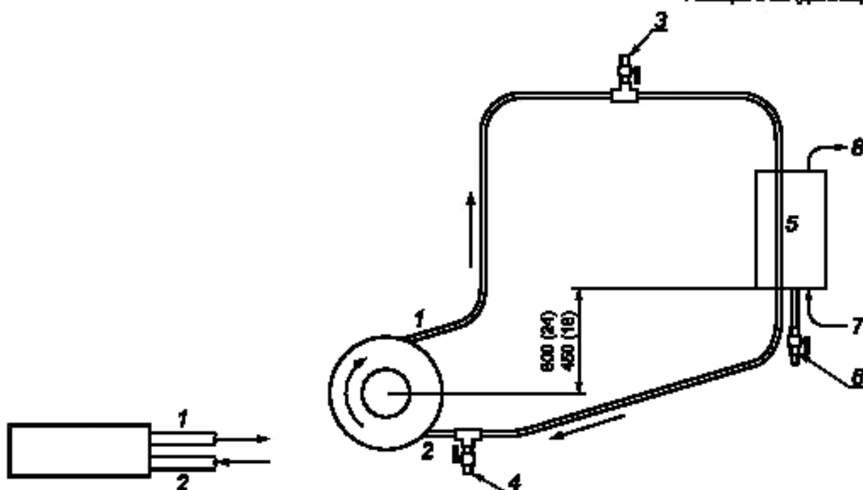
а) Конфигурация для применения с вертикальным насосом
