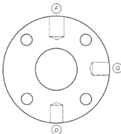
в) Типовая ориентация соединения фланца корпуса
