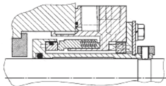
б) Альтернативное (неподвижный упругий элемент)
