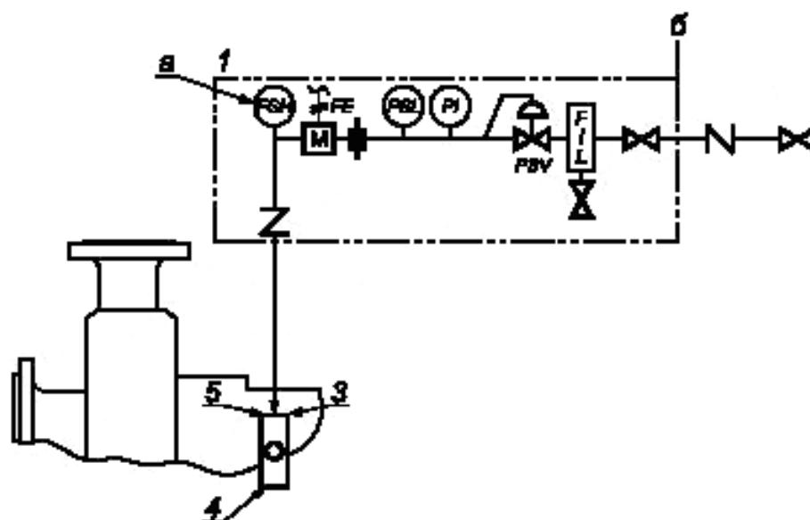
а) Трубопровод и схема измерительного прибора
