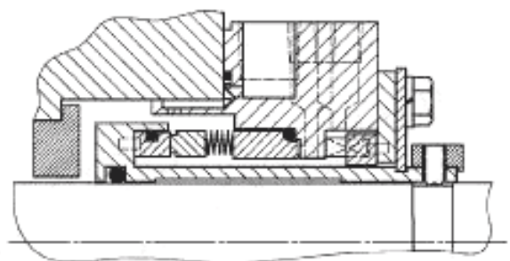
б) Альтернативное (неподвижный узел сифона)
