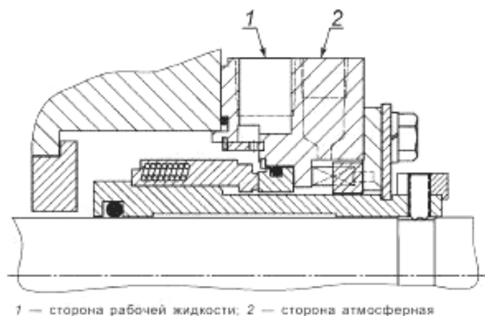
Рисунок 16 — Соединения системы трубопроводов торцового уплотнения
