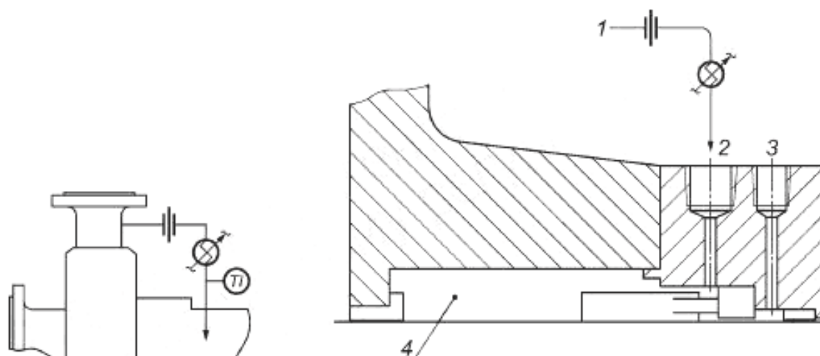
а) Трубопровод и схема измерительного прибора
