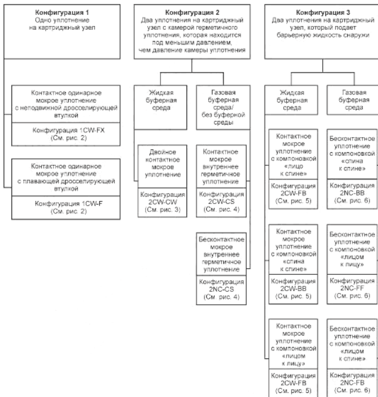
Рисунок 1 — Конфигурация уплотнения
