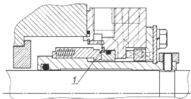
1 — удерживающая деталь (в соответствии с 6.1.1.11)
