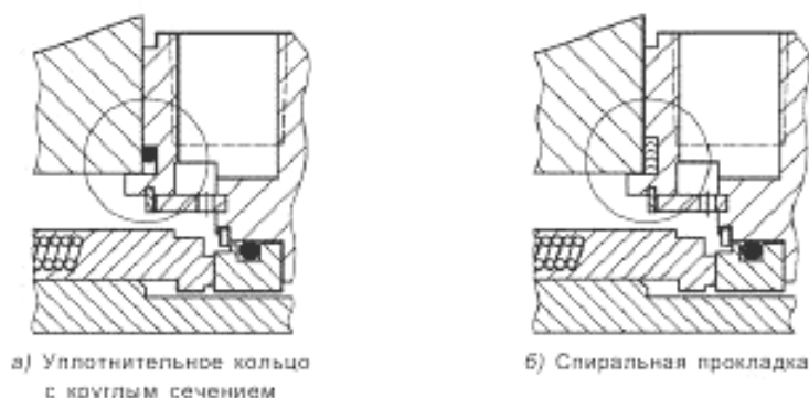
Рисунок 23 — Сопряженные соединения уплотнений
