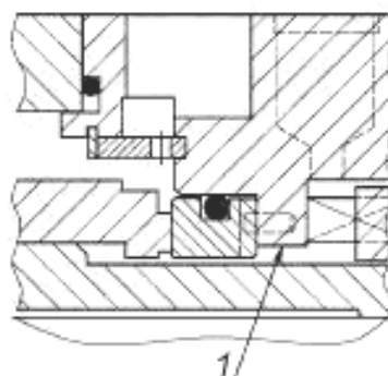
1 — выступ фланца корпуса
