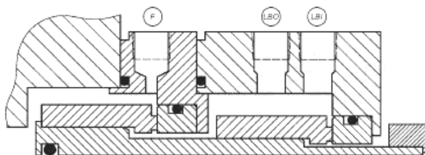
а) 2CW-CW, сдвоенное контактное жидкостное уплотнение
