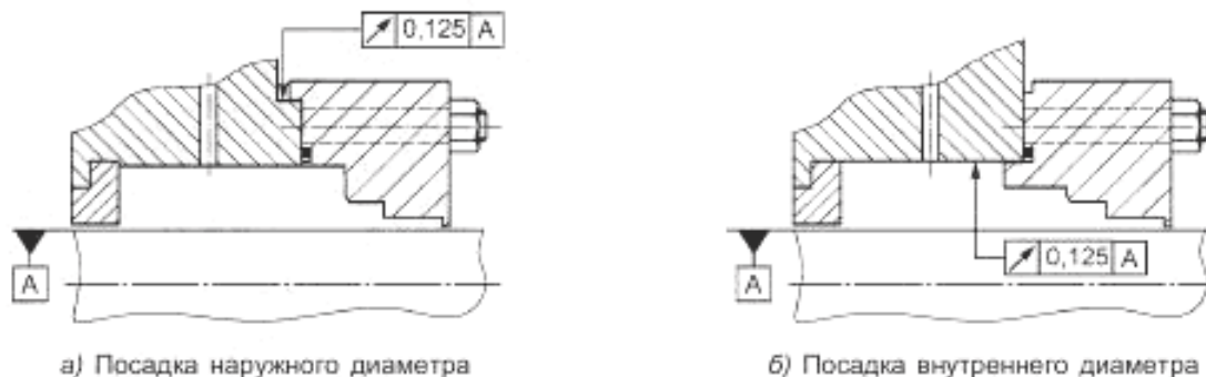
Рисунок 13 — Зарегистрированная соосность камеры уплотнения
