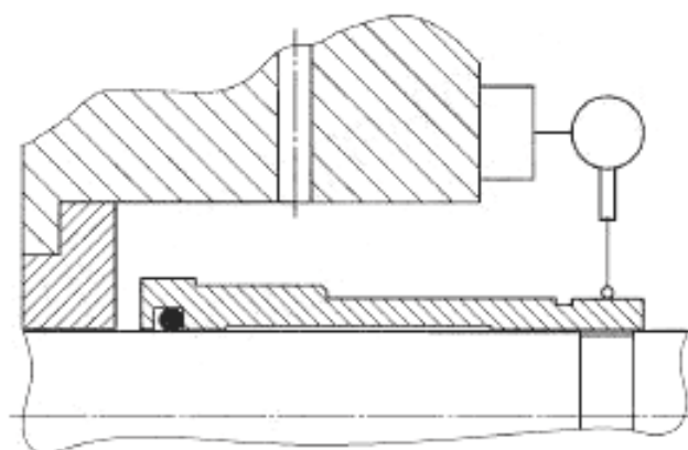
Рисунок 18 — Биение втулки уплотнения
