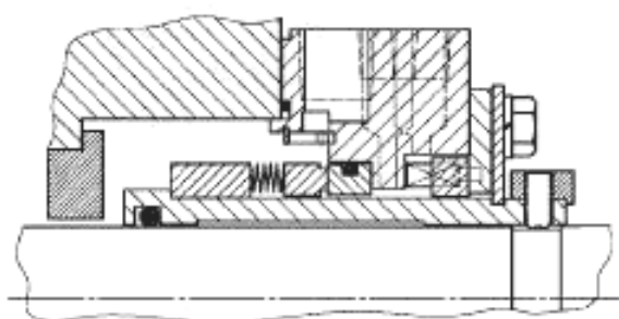
а) Стандартное (вращающийся узел сифона)
