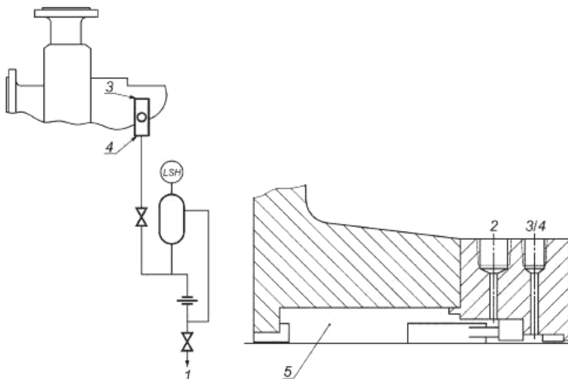
а) Трубопровод и схема измерительного прибора
