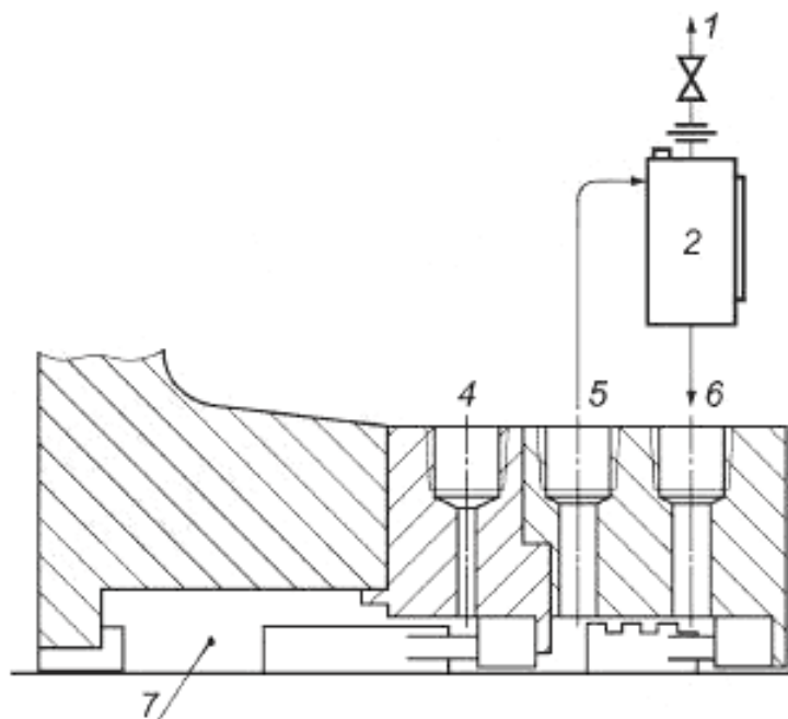
б) Детали камеры уплотнения
