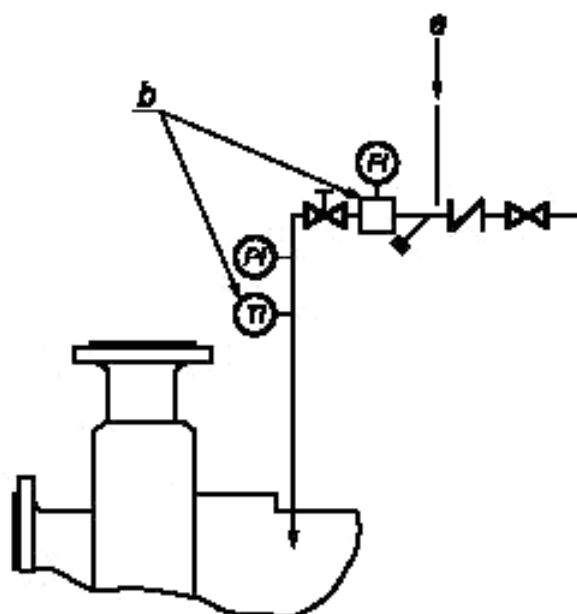
а) Трубопровод и схема измерительного прибора
