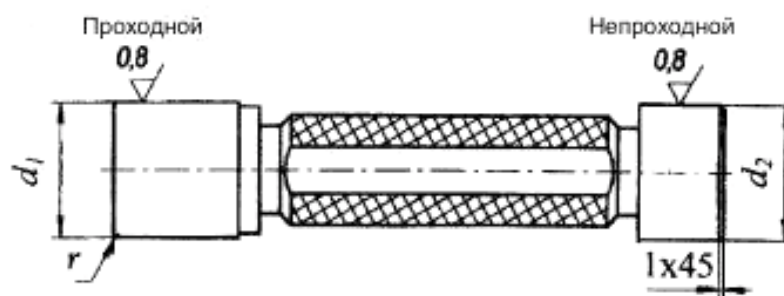
Рисунок А.2 – Проходные и непроходные калибры-пробки для контроля охватывающих концов фитингов
