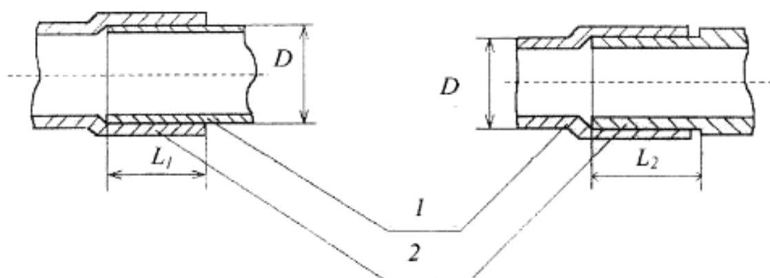
1 – труба; 2 – фитинг; D – диаметр соединяемых труб; L_1 – длина внутреннего участка под пайку для фитинга, охватывающего трубу в соединении; L_2 – длина наружного участка под пайку для фитинга, охватываемого трубой в соединении.
