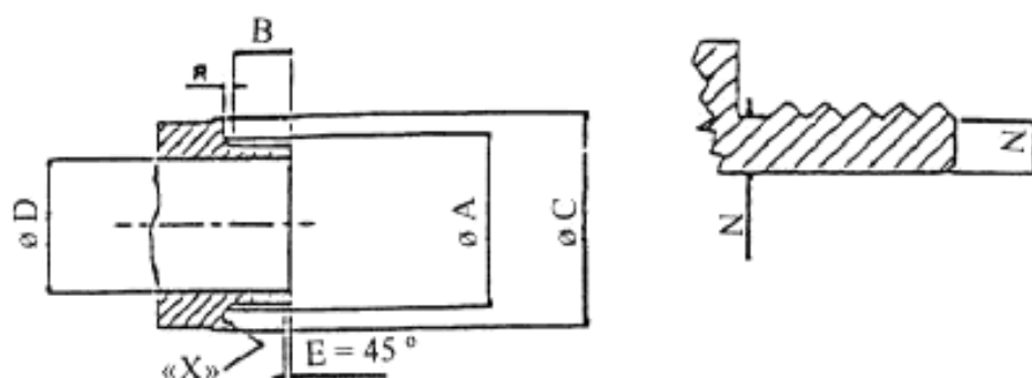
Рисунок 5 – Наружное цилиндрическое резьбовое соединение по ГОСТ 6357
