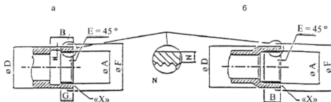
Рисунок 1 — Внутреннее цилиндрическое резьбовое соединение с резьбой по ГОСТ 6357
