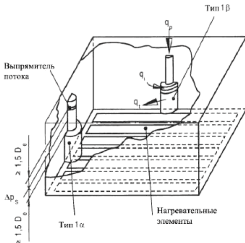
Рисунок 1 - Испытательный стенд для устройств типа 1
