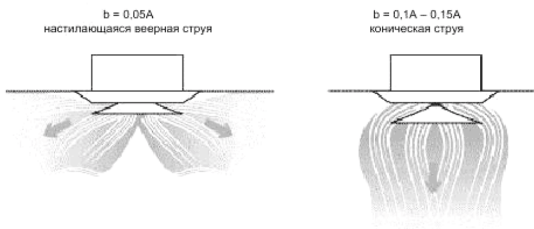
Рисунок 2 – Схемы струй, формируемых диффузором
