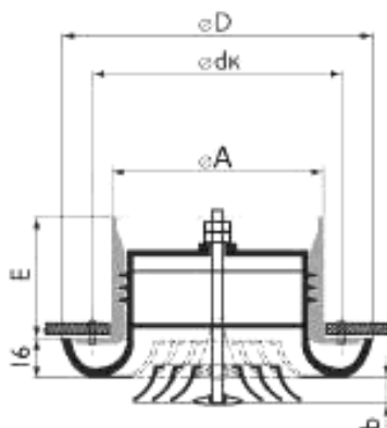
Рисунок 1 – Конструктивная схема диффузора веерного
