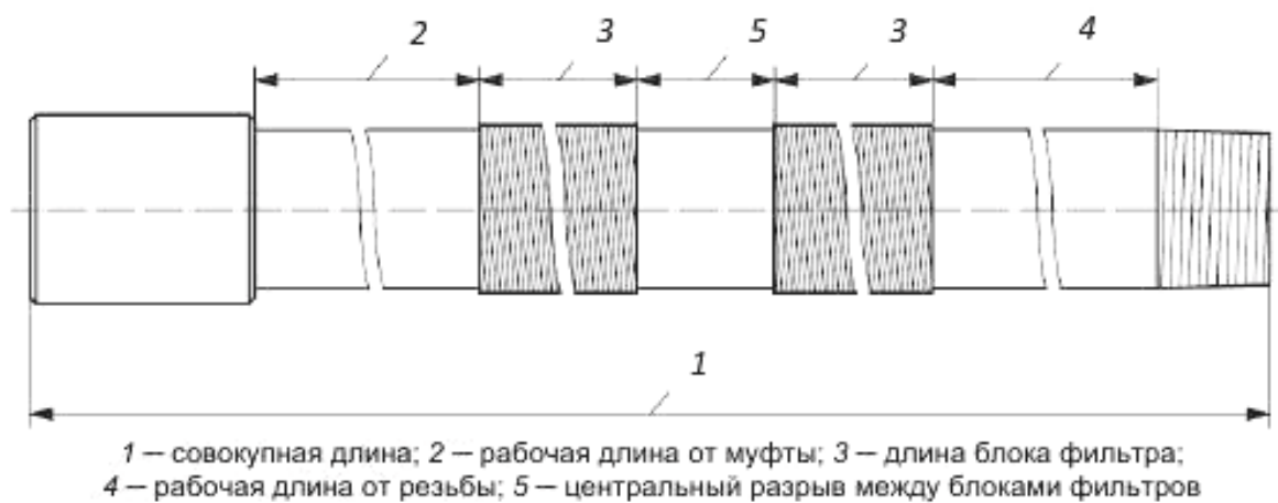
Рисунок D.3 — Комплект с двумя противопесочными фильтрами
