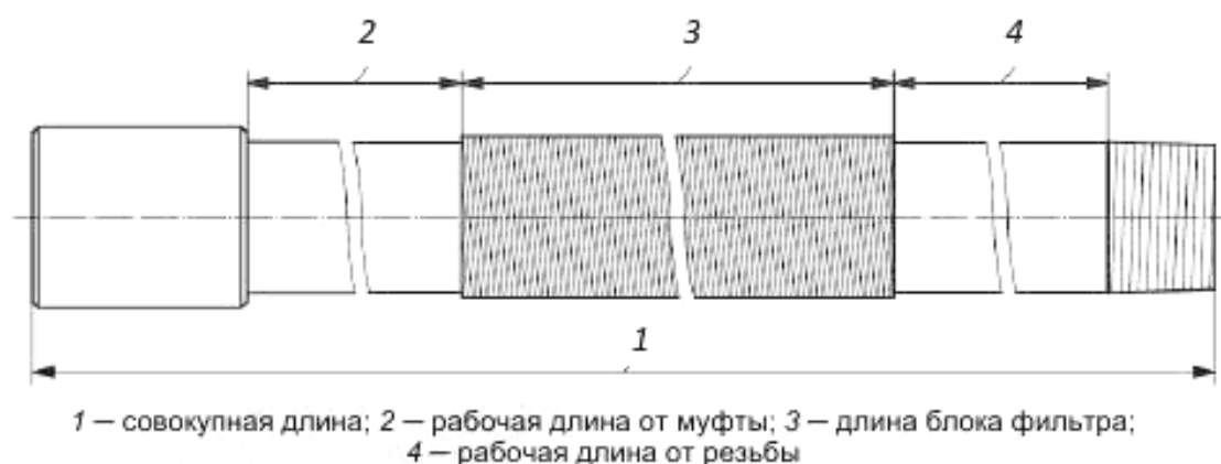
Рисунок D.2 — Комплект с одним противопесочным фильтром
