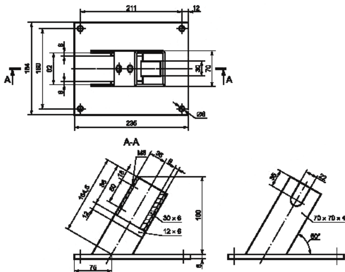
Рисунок 8 — Опорный стенд
