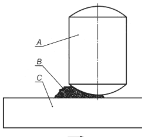
Рисунок 18 — Фарфоровая пластина и шпindel
