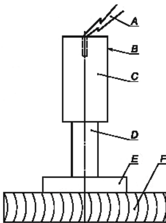
А — электрический детонатор; В — контейнер из тонкого картона (диаметр 8,6 см, длина 16,2 см); С — образец взрывчатой химической продукции; D — свинцовый цилиндр; E — стальная плита (15 × 15 × 2,5 см); F — деревянный брусок (30 × 30 × 5 см)
