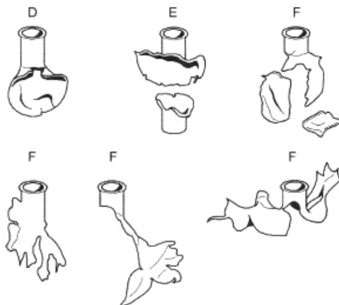
Рисунок 6 — Примеры разрушений видов D, E и F
