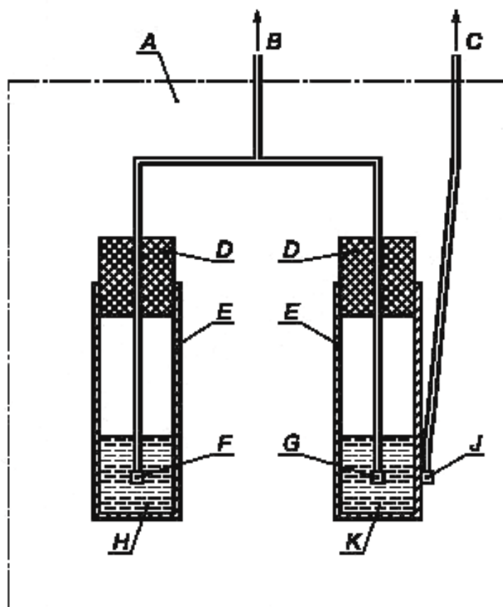
A — печь; B — к милливольтметру ( T_1 — T_2 ); C — к милливольтметру ( T_3 ); D — пробки; E — пробирки; F — термопара № 1 ( T_1 ); G — термопара № 2 ( T_2 ); H — 100 см 3 образца; J — термопара № 3 ( T_3 ); K — 100 см 3 эталонной химической продукции
