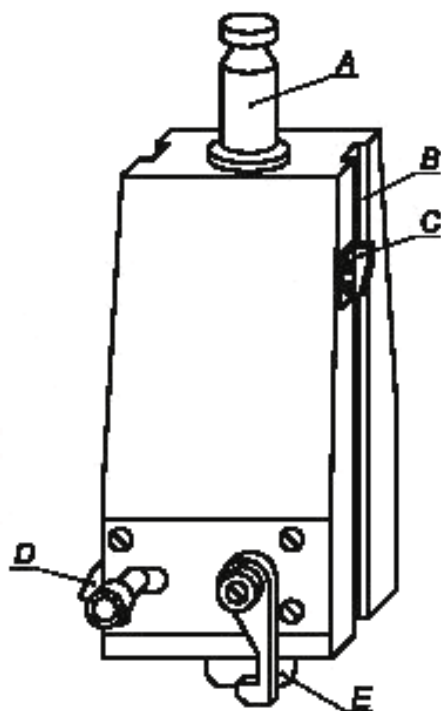
А — стержень подвески; В — направляющий паз; С — отметчик высоты; D — стопор отскока; Е — цилиндрическая ударная головка
