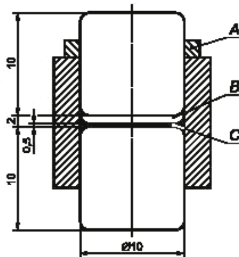
A — резиновое кольцо; B — пространство, не заполненное жидкостью; C — жидкий образец, распределенный по окружности стального цилиндра
