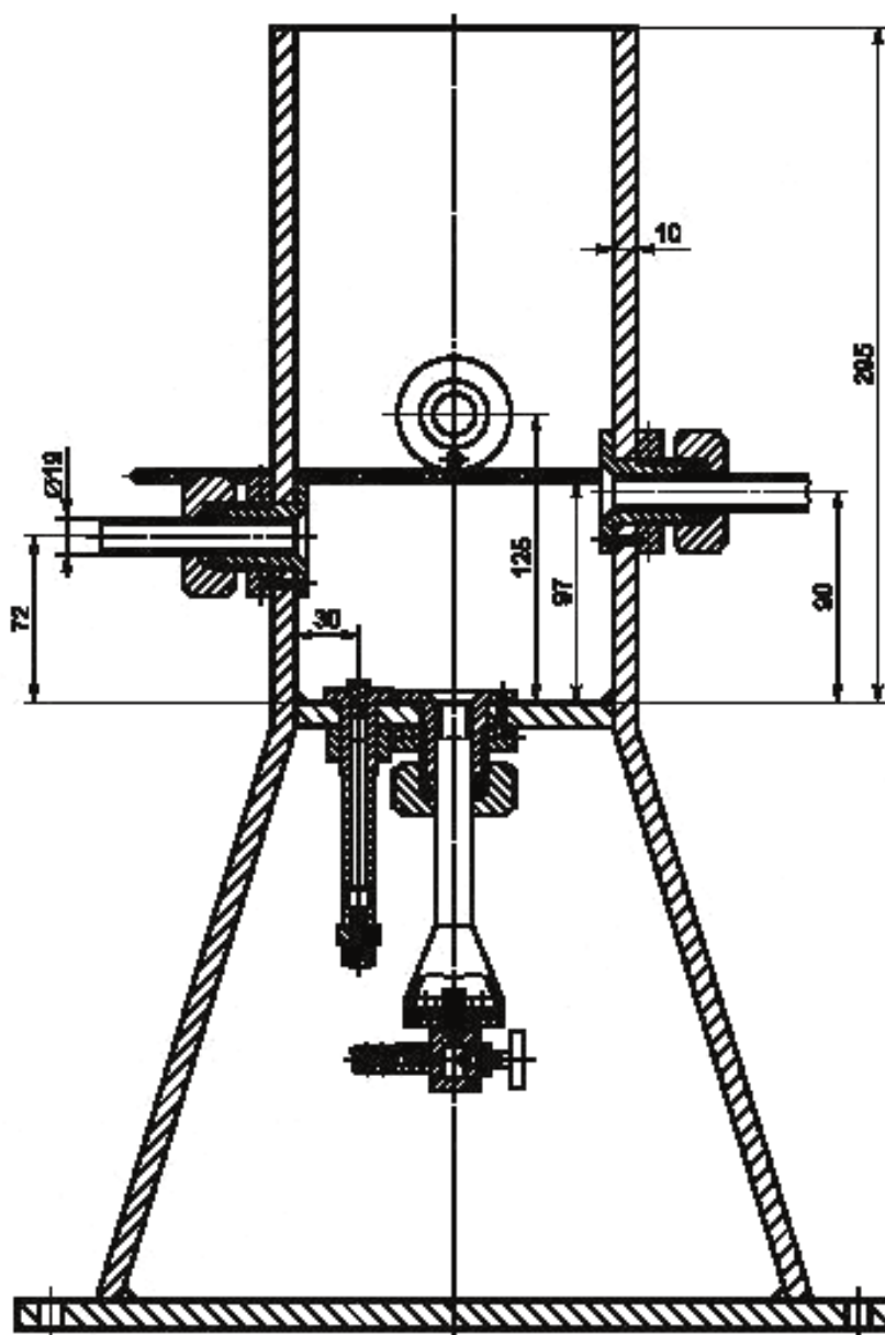
Рисунок 5 — Защитно-нагревательное устройство
