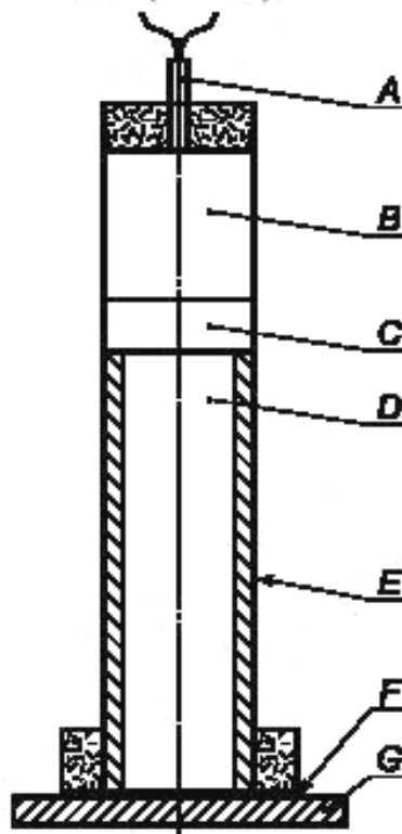
А — детонатор; В — бустерный заряд; С — прокладка из ПММА; D — испытуемая химическая продукция; E — стальная трубка; F — воздушный зазор; G — контрольная пластина
