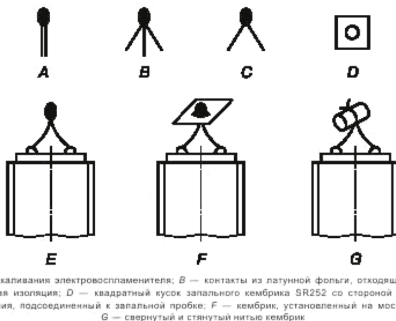
Рисунок 9 — Система зажигания для твердой химической продукции
