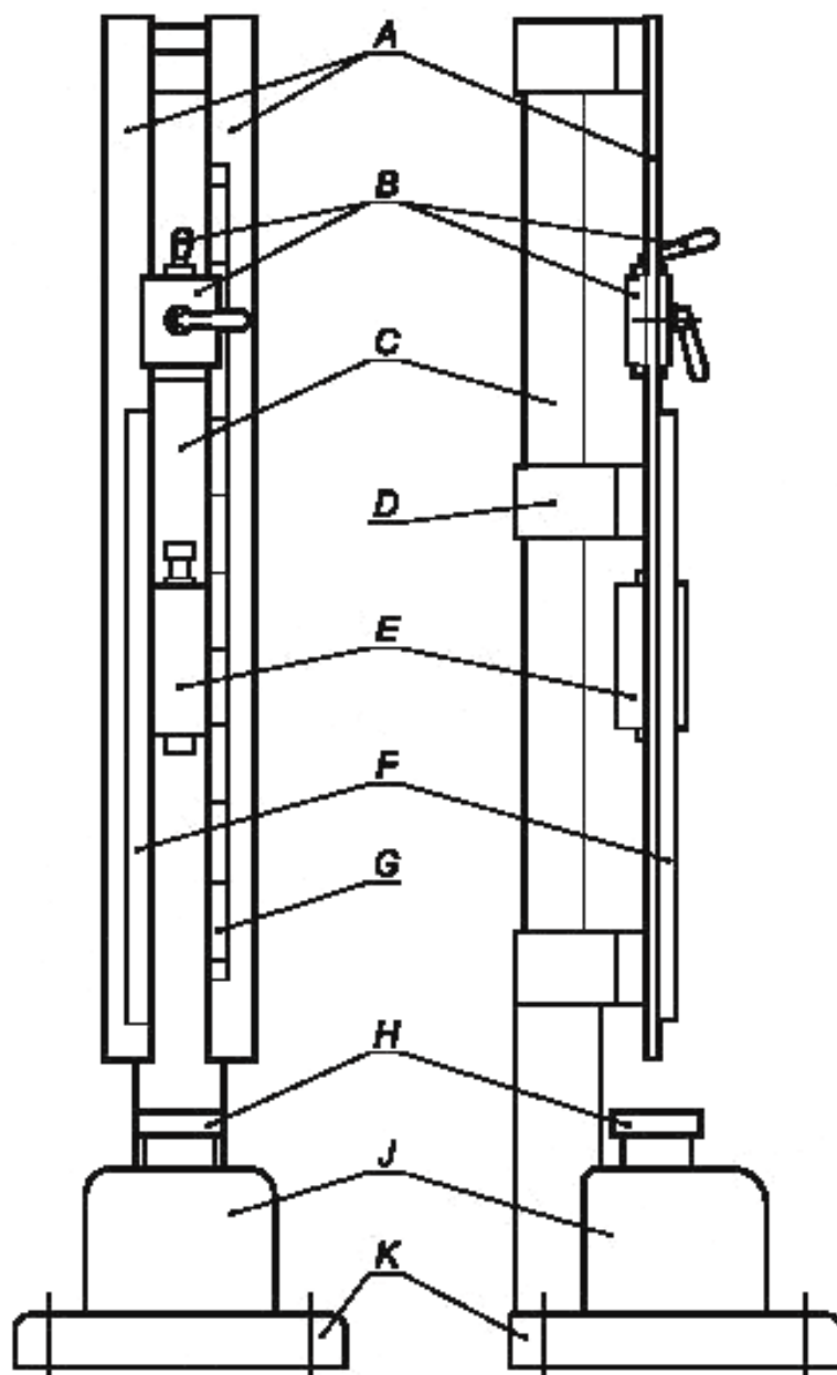
А — две направляющие рейки; В — захватно-пусковое устройство; С — стойка; D — средняя перекладина; Е — падающий груз; F — зубчатая рейка; G — градуированная шкала; H — наковальня ( \varnothing 100 \times 70 мм); J — стальной блок, 230 \times 250 \times 200 мм; K — основание, 450 \times 450 \times 60 мм
