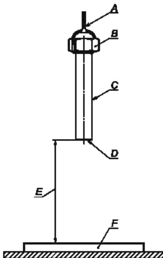
А — шнур; В — чугу́нный ко́лпачок с резьбой; С — бесшовная стальная труба; D — сварная стальная основа (толщиной 4 мм); E — высота падения (0,25 — 5 м); F — стальная наковальня (1 × 0,5 м, толщина — 0,15 м)
