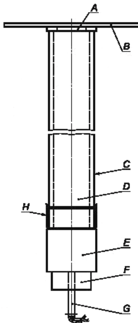
А — прокладки; В — контрольная пластина; С — стальная трубка; D — испытуемая химическая продукция; E — бустер, состоящий из циклотриметилентринитрамина/парафина или ТЭН/тротила; F — держатель детонатора; G — детонатор; H — пластмассовая мембрана
