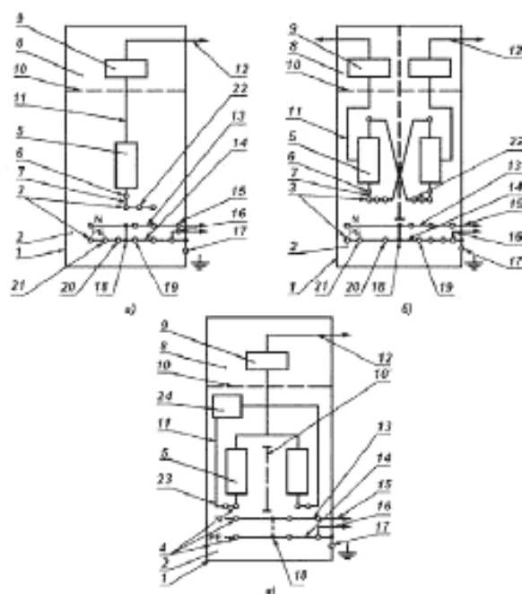
а) с одним вводом; б) с двумя вводами; в) с двумя взаиморезервируемыми вводами с аппаратурой АВР
