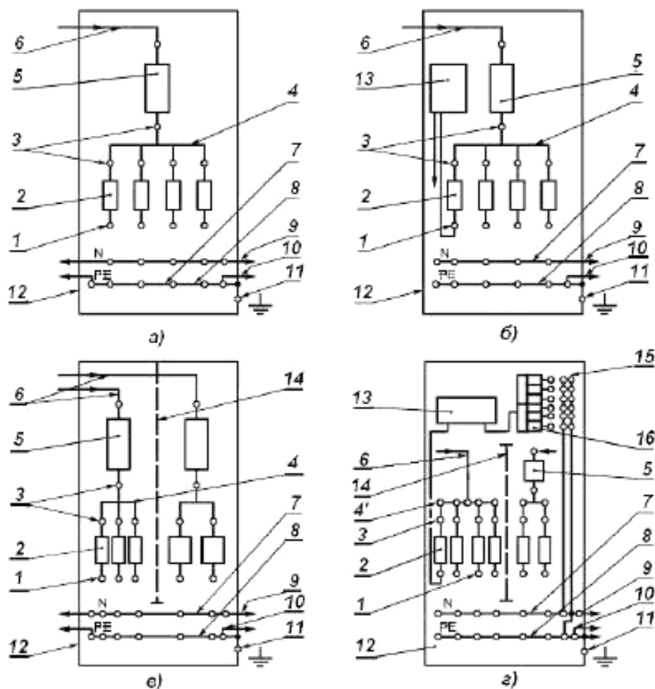
а) с блоком распределения, запитываемым от одного ввода; б) с блоками распределения и учета, запитываемыми от одного ввода; в) с блоками распределения, запитываемыми от двух вводов; г) с блоками распределения, учета и управления общедомовым освещением, запитываемыми от двух вводов
