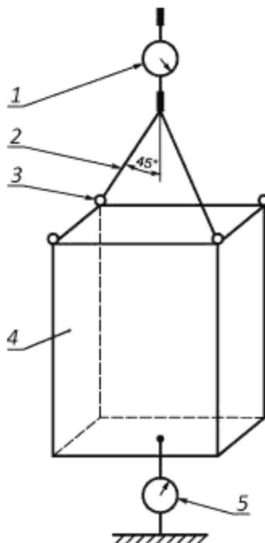
1 – динамометр 1; 2 – строп; 3 – строповое устройство; 4 – ВРУ; 5 – динамометр 2
