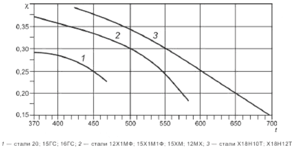
Рисунок 8.1 — Коэффициент усреднения компенсационных напряжений \chi
