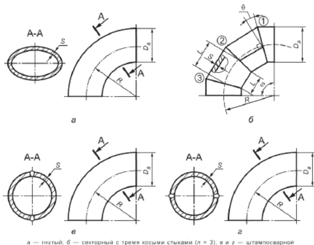
Рисунок 7.1 — Отводы
