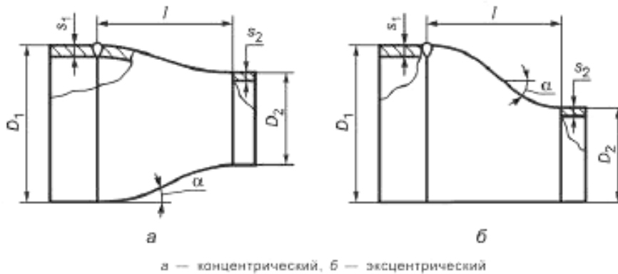
Рисунок 7.2 — Переходы
