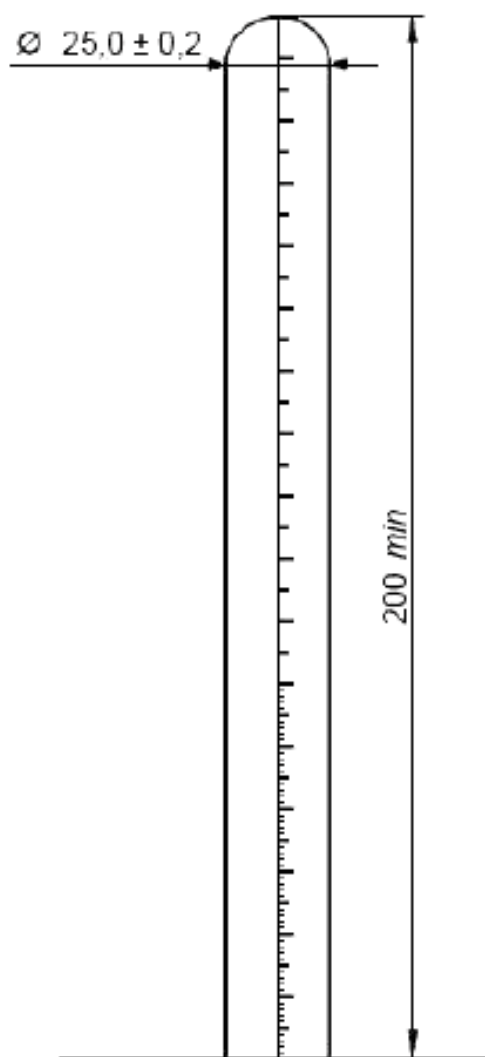
Рисунок А1.1 – Градуированный стержень для определения длины презерватива
