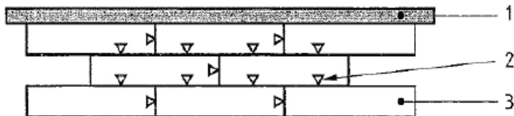
1 – поверочная линейка; 2 – точки приложения щупа индикаторного глубиномера в местах соединения элементов напольного покрытия; 3 – образец для испытания
