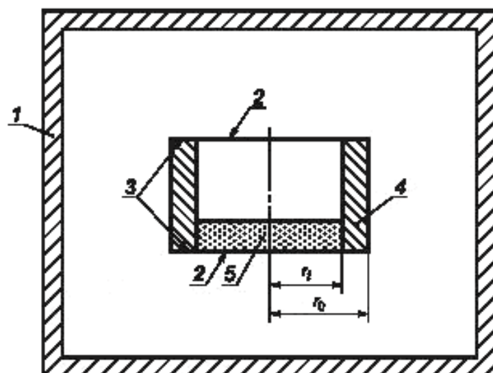
Рисунок 1 — Схема испытания по определению характеристик паропроницаемости
