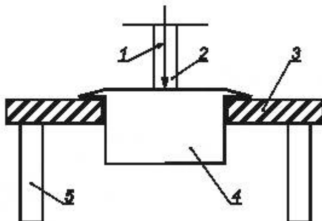
Рисунок 101 — Место приложения силы при испытании сжатием по 15.101
