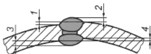
1 — наружное радиальное смещение; 2 — высота наружного валика сварного шва; 3 — высота внутреннего валика сварного шва; 4 — внутреннее радиальное смещение
