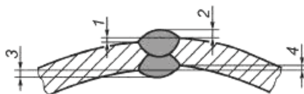
1 — наружное радиальное смещение; 2 — высота наружного валика сварного шва; 3 — высота внутреннего валика сварного шва; 4 — внутреннее радиальное смещение
