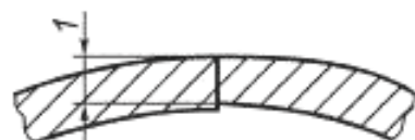
1 — остаточная толщина стенки в сварном шве
