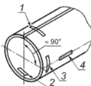
1 — L — продольная проба; 2 — T — поперечная проба a — Бесшовная труба
