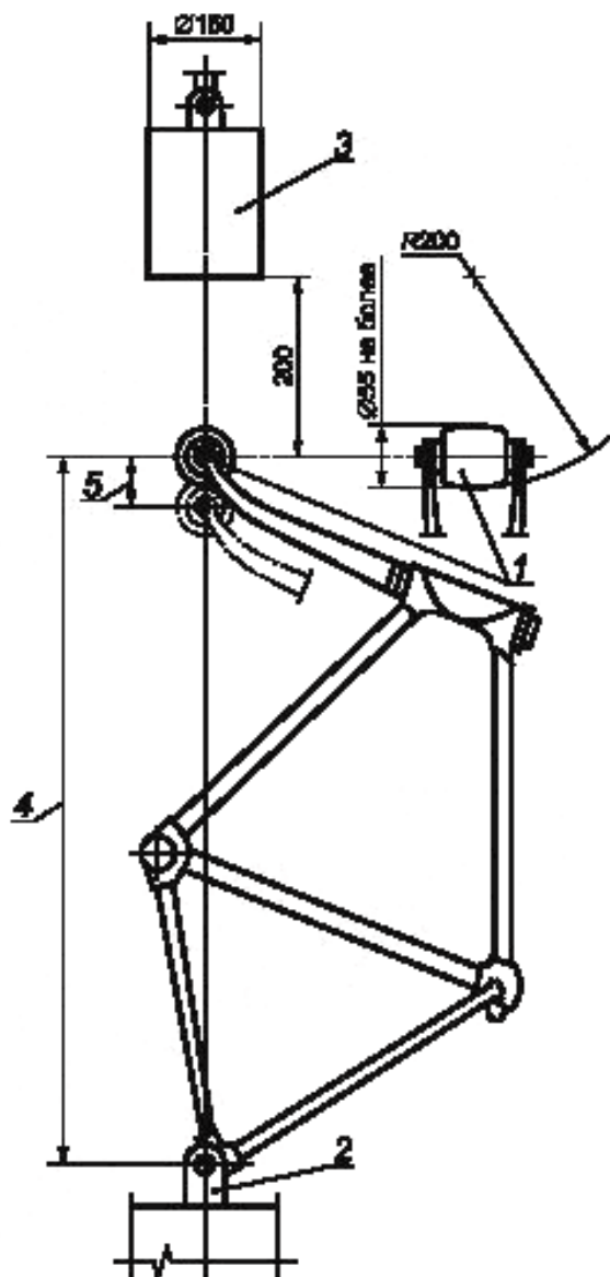
1 — ролик; 2 — зажимное приспособление; 3 — груз; 4 — база копес; 5 — остаточная деформация
