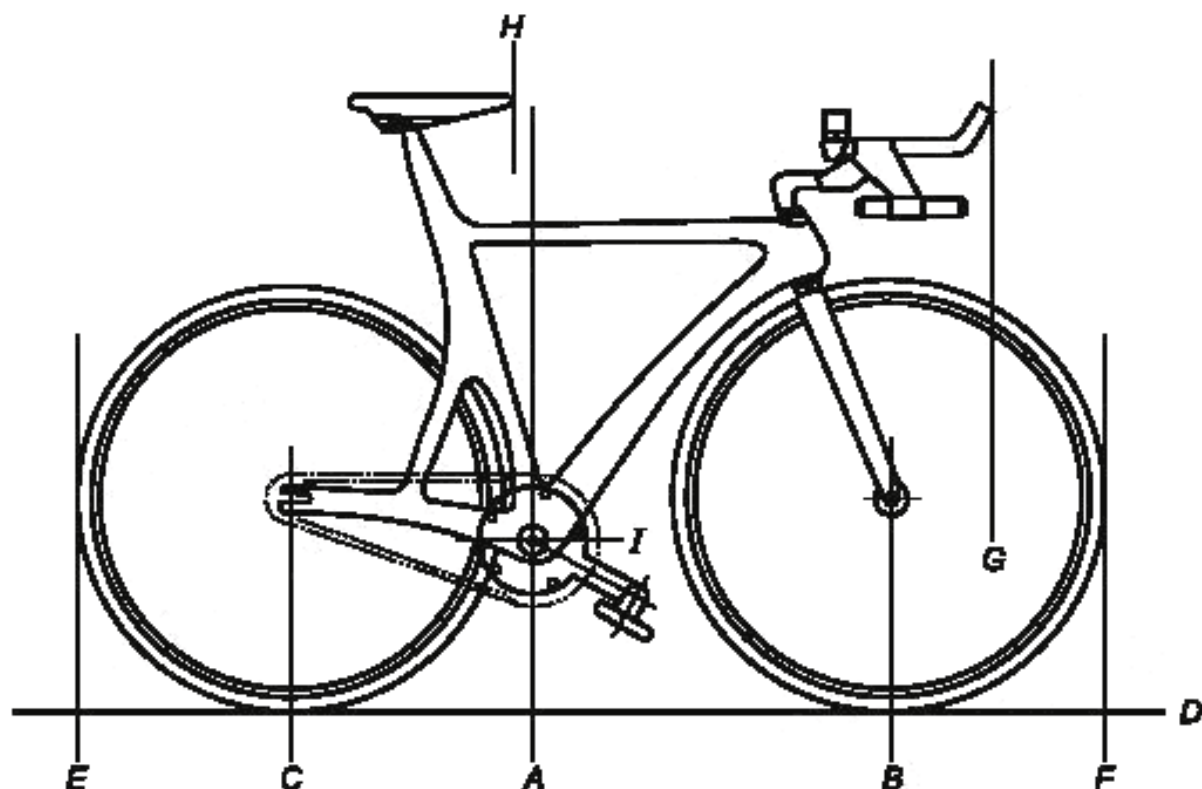
Рисунок 1 — Основные параметры и размеры велосипеда
