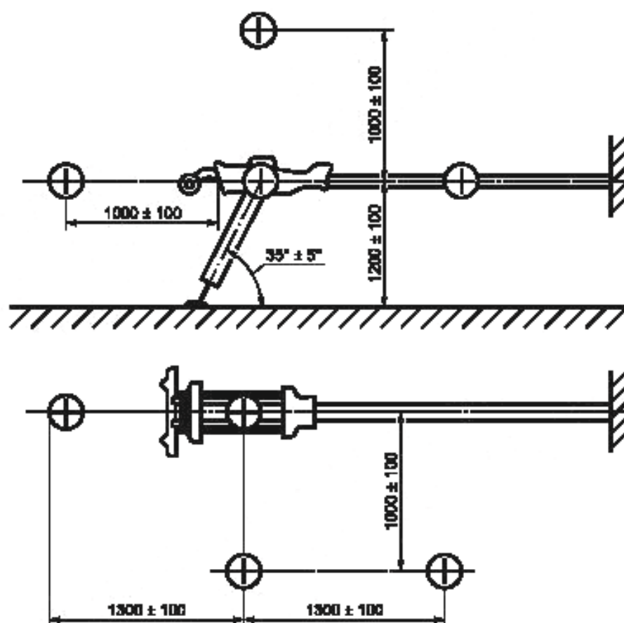
Схема установки перфоратора и точек измерения при определении шумовой характеристики перфоратора
