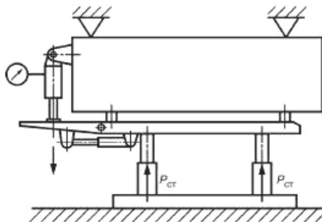
Рисунок А.2 — Схема нагружения гидродожимного козырька перекрытия
