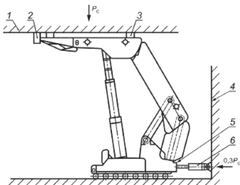
1 — нагрузочная плита; 2 — упор; 3, 5 — тензоопоры; 4 — колонна стенда; 6 — гидродомкрат
