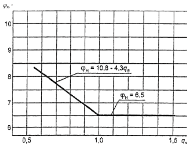
Рисунок 3 – Зависимость угла крена \varphi_n подрессоренных масс АТС от коэффициента поперечной устойчивости q_s
