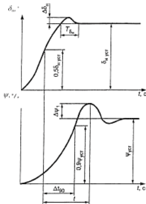
Рисунок 4 – Записи угла поворота рулевого колеса \delta_w и угловой скорости \psi автомобиля при испытании «рывок руля»
