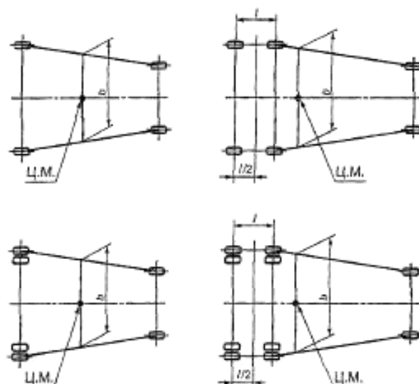
Рисунок 1 – Схемы определения величины приведенной колеи b
