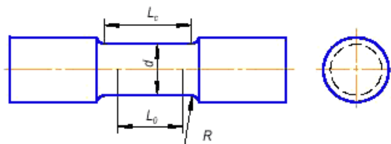
с – Цилиндрический образец
