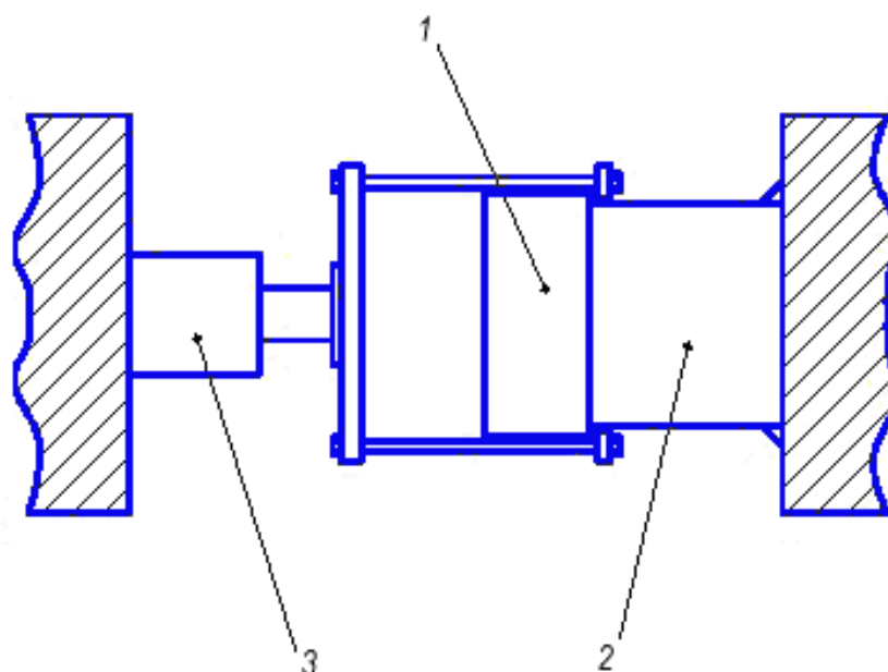
1 – резьбовая предохранительная деталь; 2 – участок трубы; 3 – гидроцилиндр
