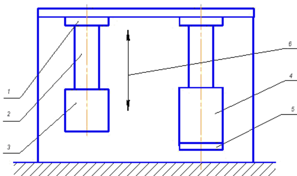
1 – испытательный стенд; 2 – ниппельный конец трубы; 3 – ниппельная предохранительная деталь; 4 – муфта; 5 – муфтовая предохранительная деталь; 6 – направления движения
