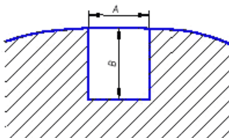
b – Надрез на наружной поверхности
