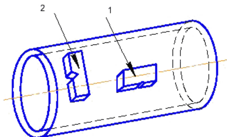
1 – продольный образец; 2 – поперечный образец.
