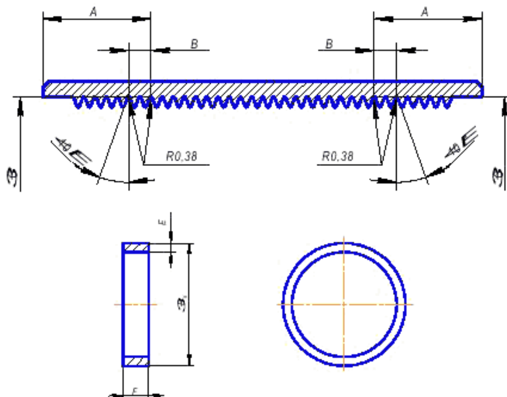
Рисунок D.21 – SR13 Муфта с проточками под уплотнительные кольца и неметаллическое кольцо для насосно-компрессорных труб для соединений NU и НКТ
