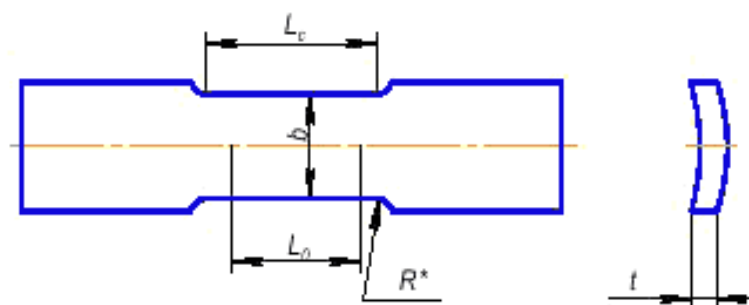
б – Образец в виде полосы*
