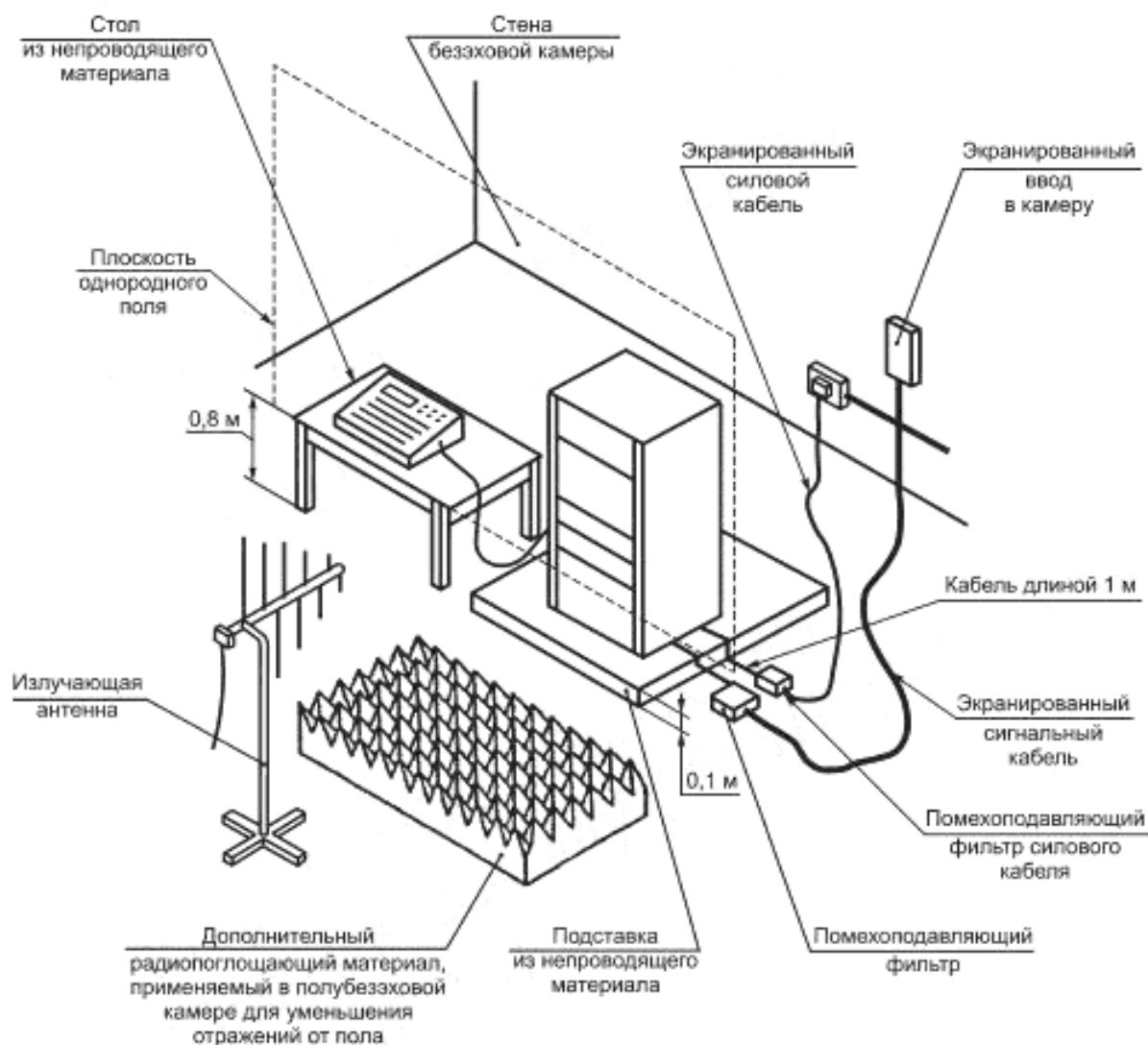
Рисунок 5 — Пример установки для испытаний напольных ТЧ
