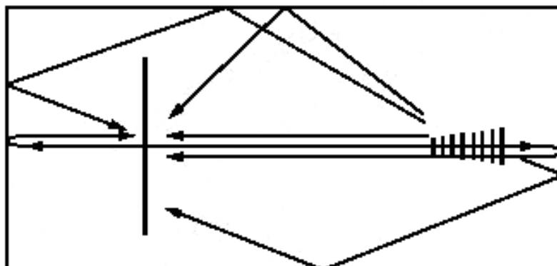
Рисунок С.1 — Многократные отражения в существующих малых беззховых камерах
