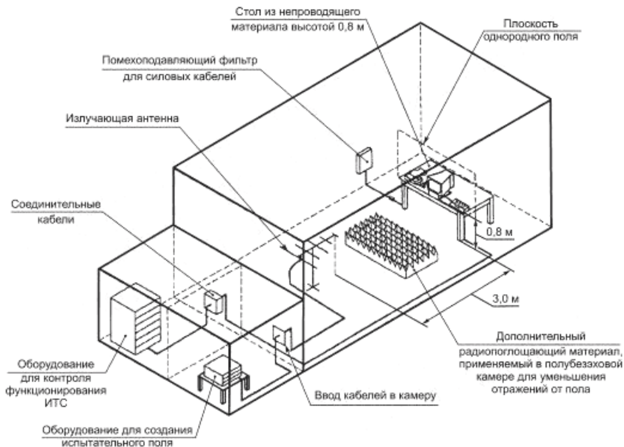
Рисунок 2 — Пример испытательной установки
