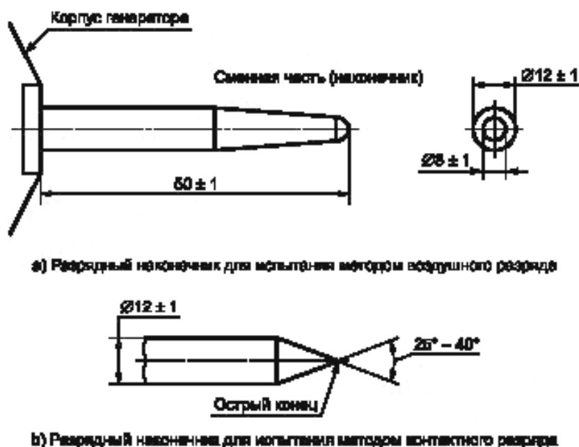
Рисунок 3 – Разрядные наконечники испытательного генератора
