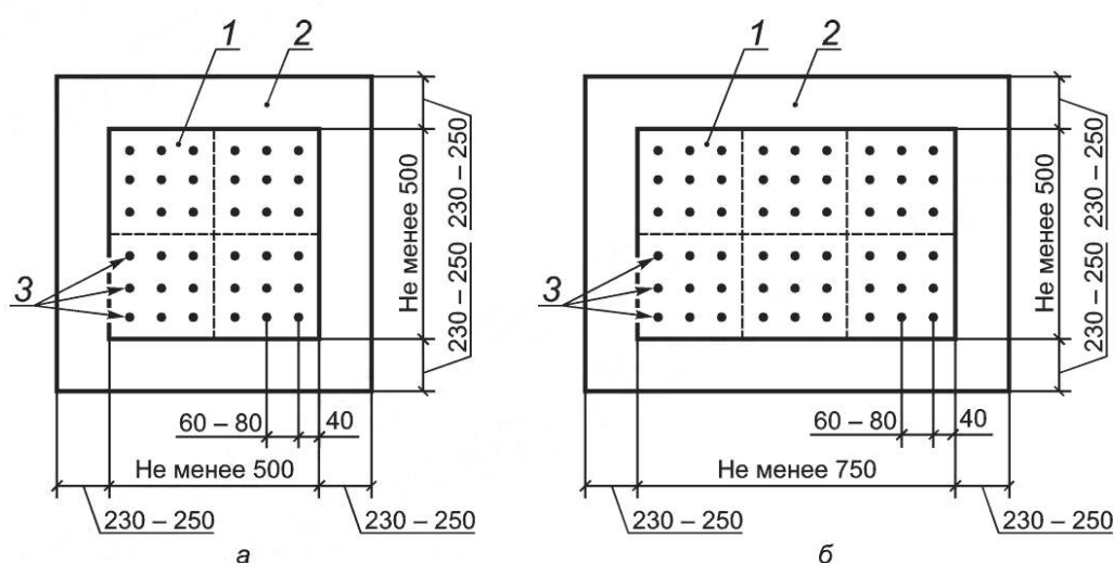
Рисунок 2 — Схема расположения точек ударов на участках пола из однородного материала (а) и из неоднородного материала (б)
