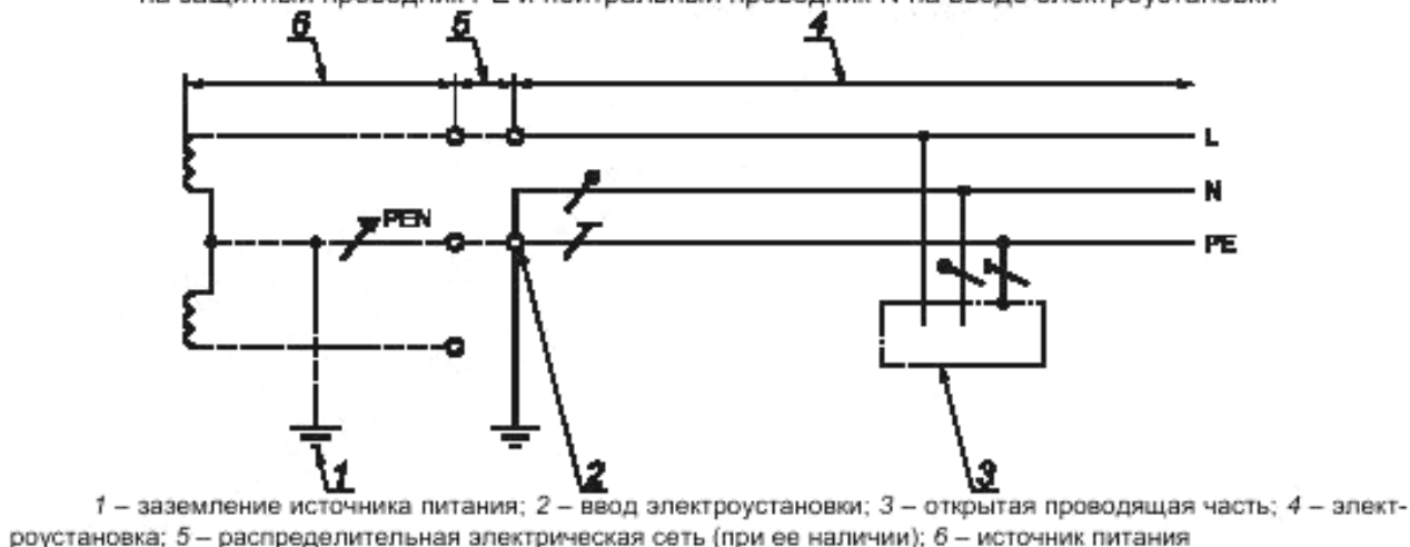
Рисунок 31B2 – Система TN-C-S трехфазная четырехпроводная, в которой PEN-проводник разделен на защитный проводник PE и нейтральный проводник N на вводе электроустановки
