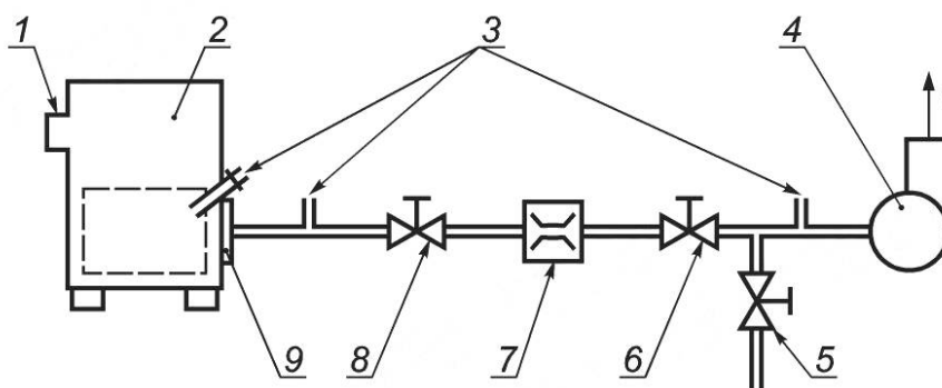
1 — выход газохода; 2 — испытуемый котел; 3 — точки измерения давления/тяги; 4 — вентилятор; 5 — вентиль 3 (перепускной); 6 — вентиль 2; 7 — расходомер; 8 — вентиль 1 (регулирующий); 9 — пластина горелки
