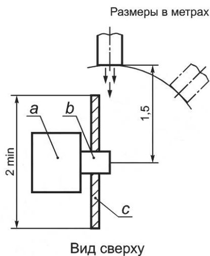
Рисунок В.1 — Расположение генератора потока воздуха для испытания с низколежащим отводящим газоходом
