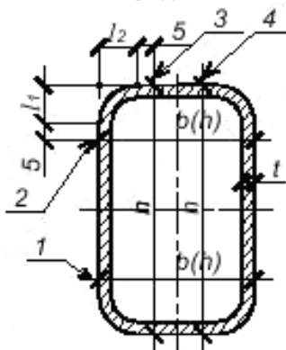
Рисунок 3 – Схема измерения размеров квадратных и прямоугольных профилей
